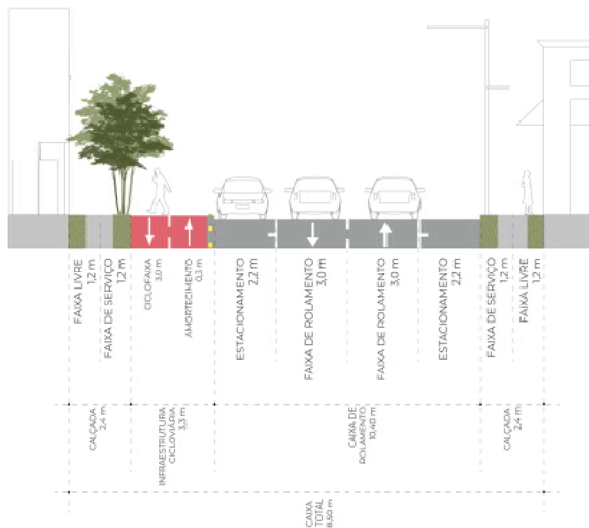
Via Coletora 2 com ciclofaixa bidirecional
