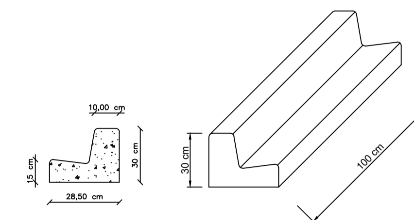
DETALHE MEIO FIO Esc. 1/20
