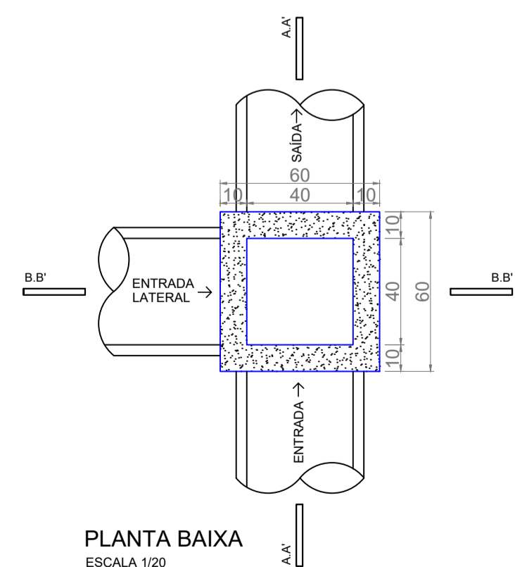
DETALHE BOCA DE LOBO
