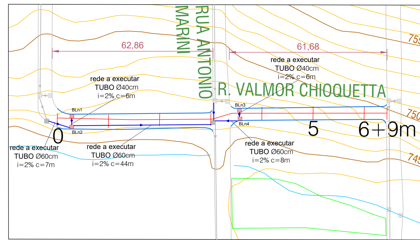
DRENAGEM - RUA VALMOR CHIOQUETTA Esc. 1/750
