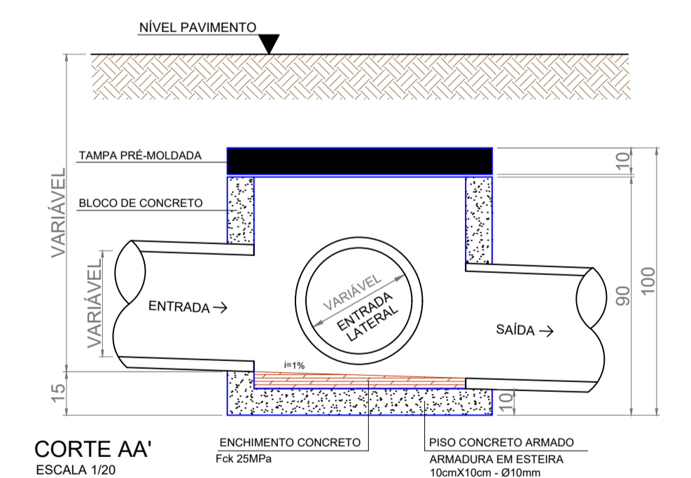
DETALHE CAIXA DE PASSAGEM
