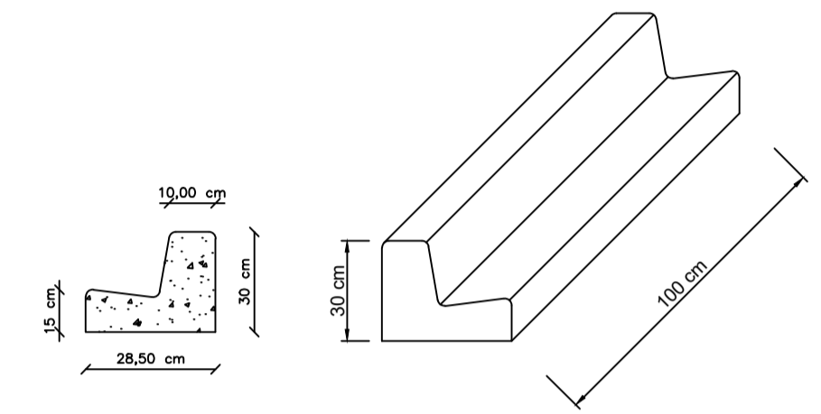
DETALHE MEIO FIO Esc. 1/20
