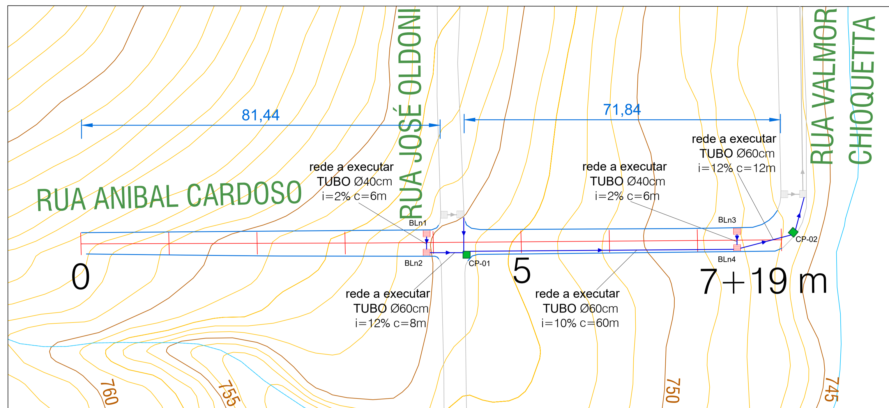
DRENAGEM - RUA ANÍBAL CARDOSO - Trecho 1 Esc. 1/500
