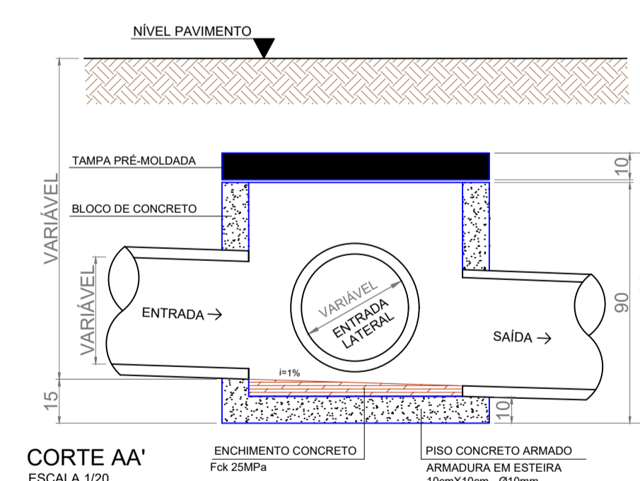
DETALHE CAIXA DE PASSAGEM
