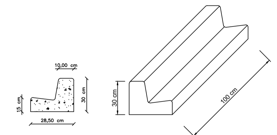
DETALHE MEIO FIO Esc. 1/20
