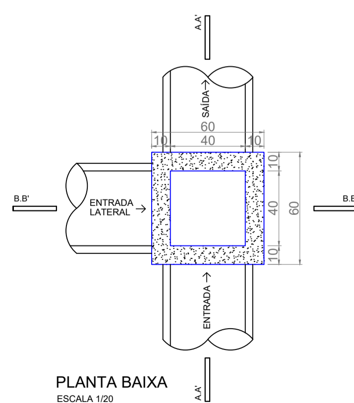
DETALHE BOCA DE LOBO
