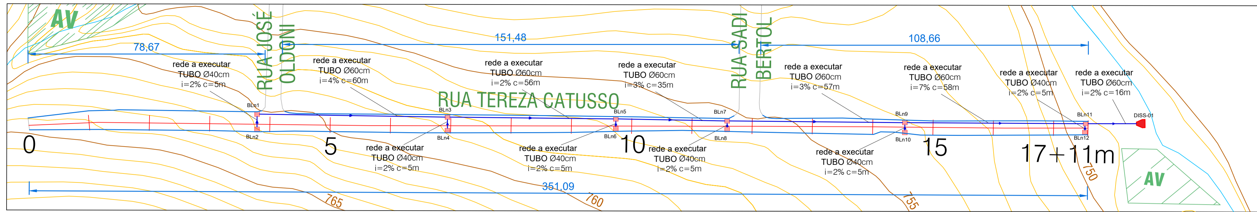
DRENAGEM - RUA TEREZA CATUSSO Esc. 1/750
