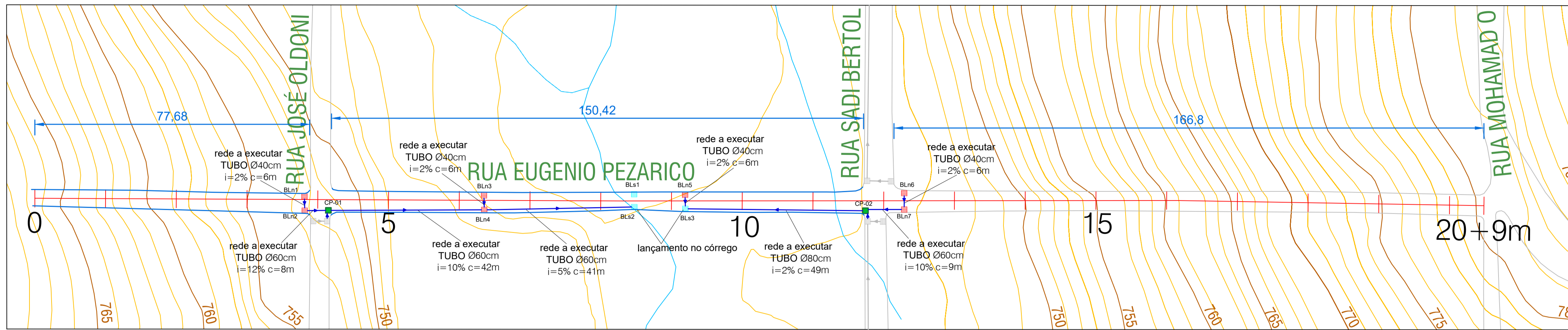
DRENAGEM - RUA EUGÊNIO PEZARICO Esc. 1/750
