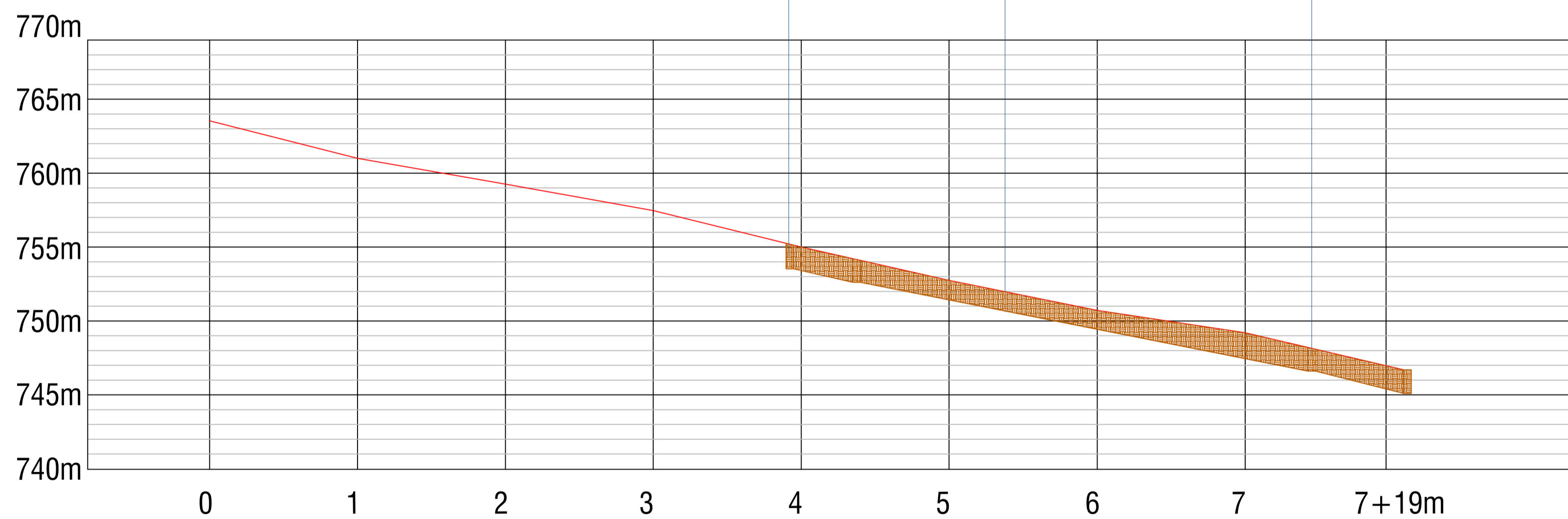
PERFIL LONGITUDINAL - RUA ANÍBAL CARDOSO - Trecho 1 Esc. 1/500
