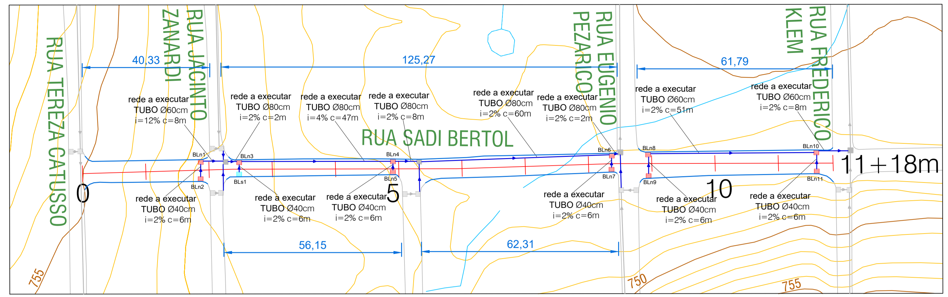
DRENAGEM - RUA SADI BERTOL Esc. 1/750
