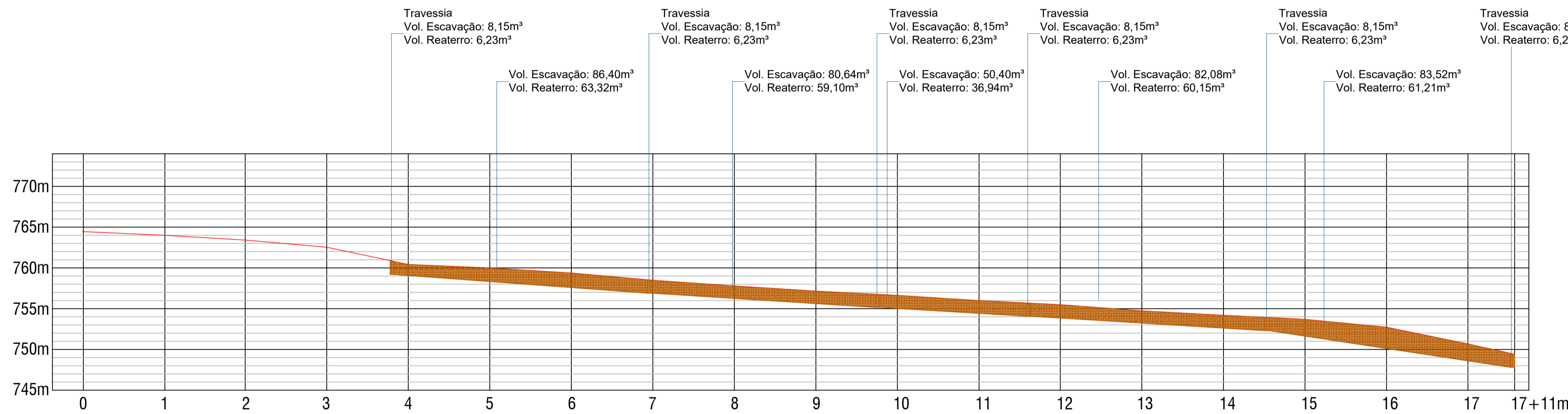
PERFIL LONGITUDINAL - RUA TEREZA CATUSSO Esc. 1/750
