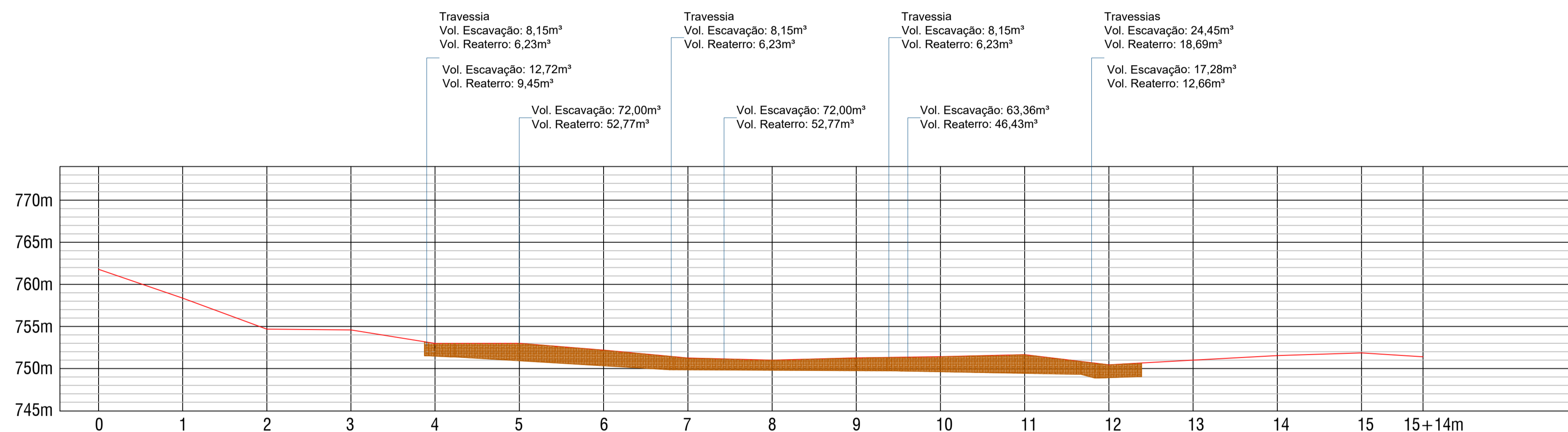
PERFIL LONGITUDINAL - RUA JACINTO ZANARDI Esc. 1/750
