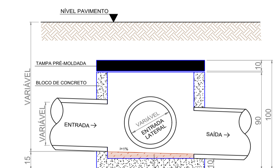
CORTE AA' ESCALA 1/20
