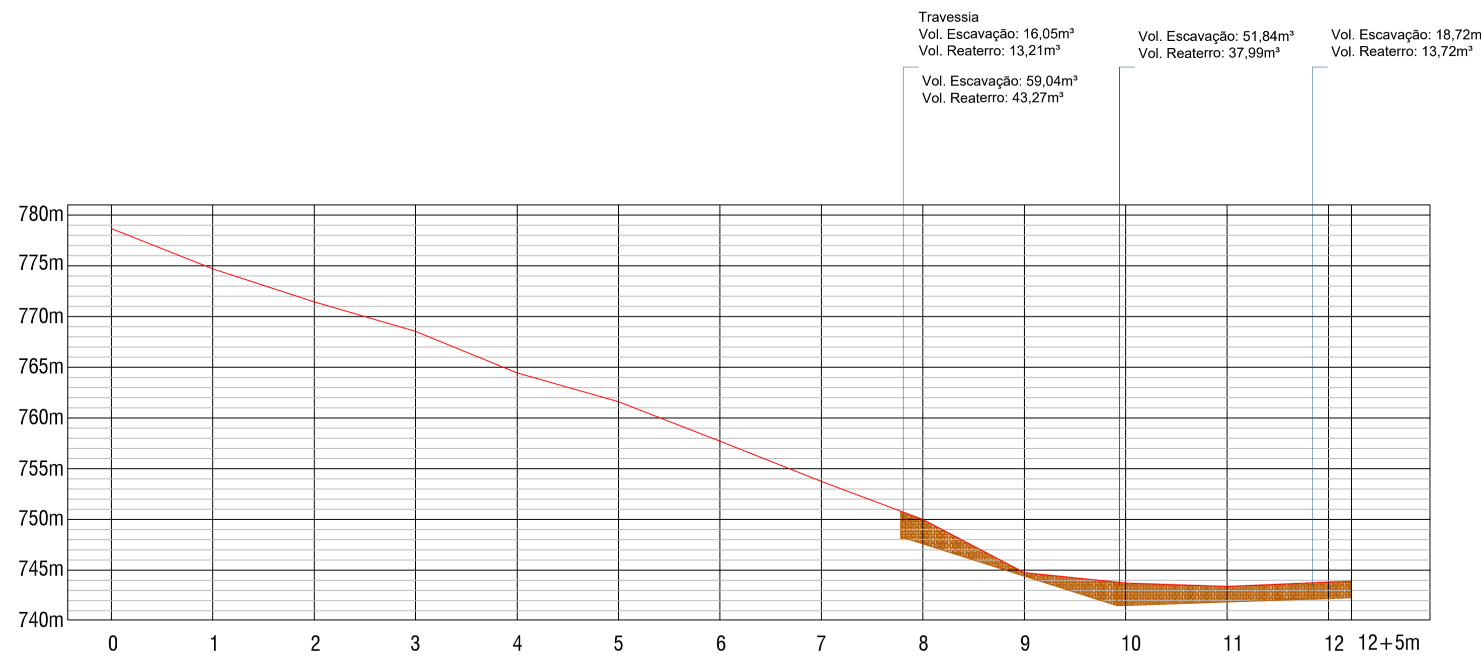
PERFIL LONGITUDINAL - RUA CLARICE RECALCATTI Esc. 1/750
