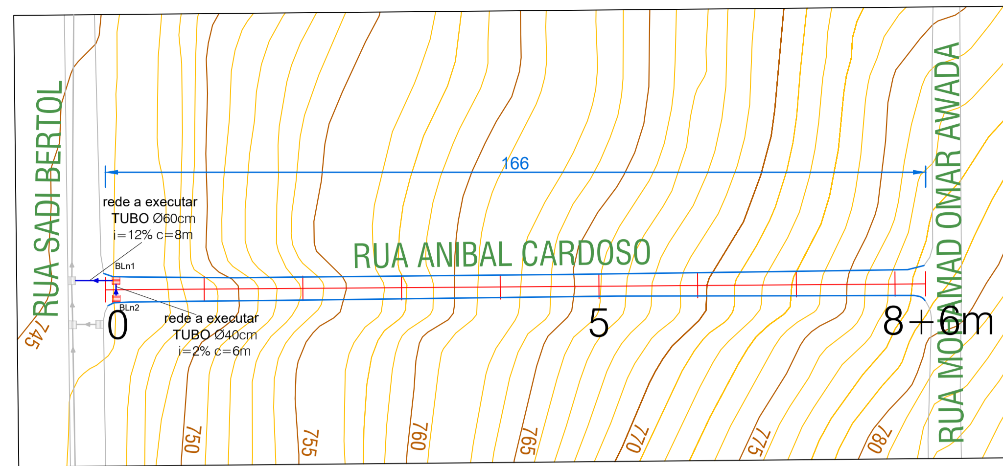
DRENAGEM - RUA ANÍBAL CARDOSO - Trecho 2 Esc. 1/750
