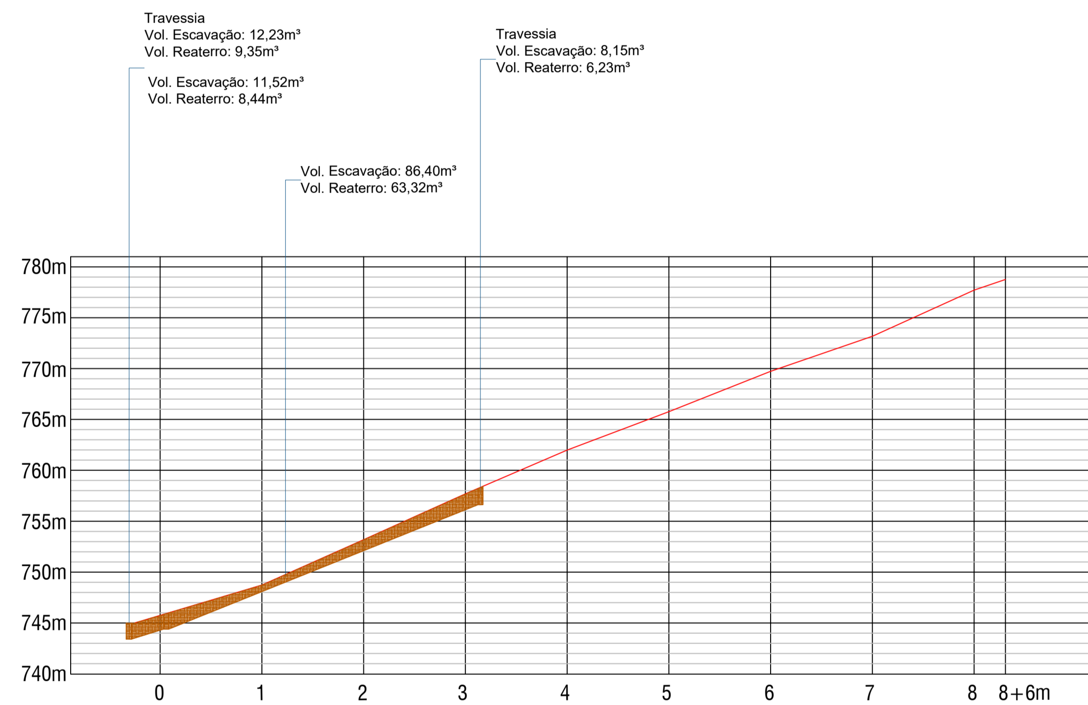
PERFIL LONGITUDINAL - RUA ANÍBAL CARDOSO - Trecho2 Esc. 1/750
