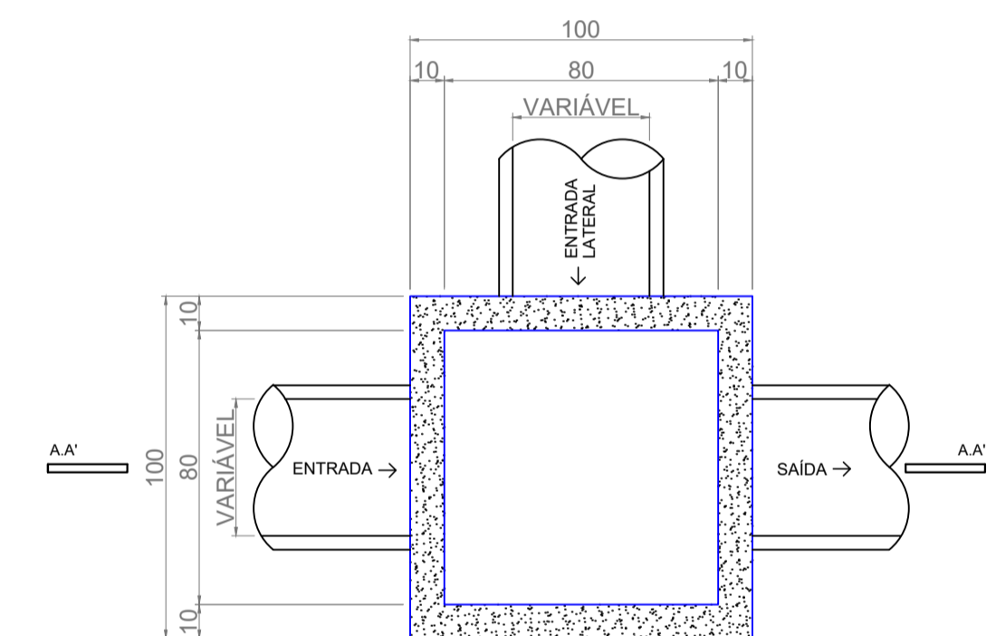
PLANTA BAIXA ESCALA 1/20
