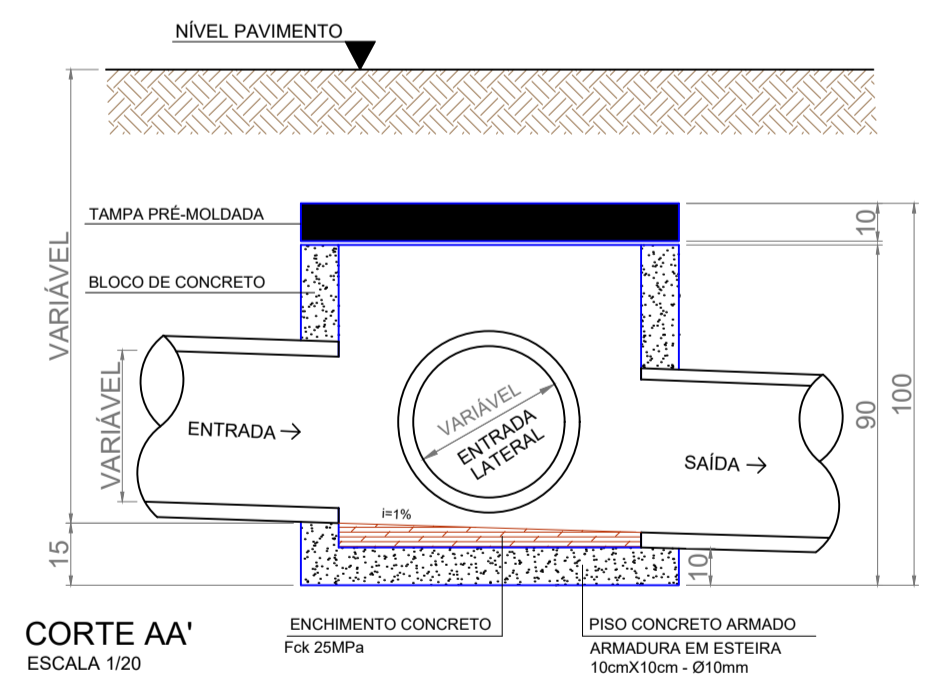
DETALHE CAIXA DE PASSAGEM
