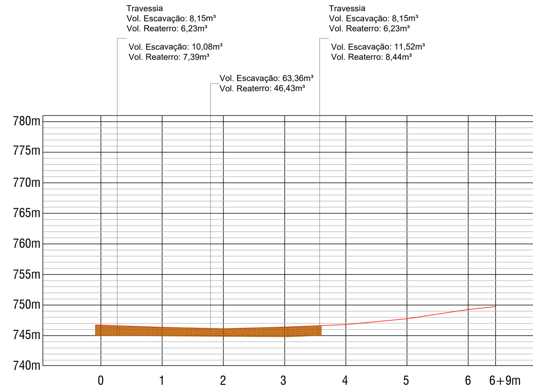
PERFIL LONGITUDINAL - RUA VALMOR CHIOQUETTA Esc. 1/750
