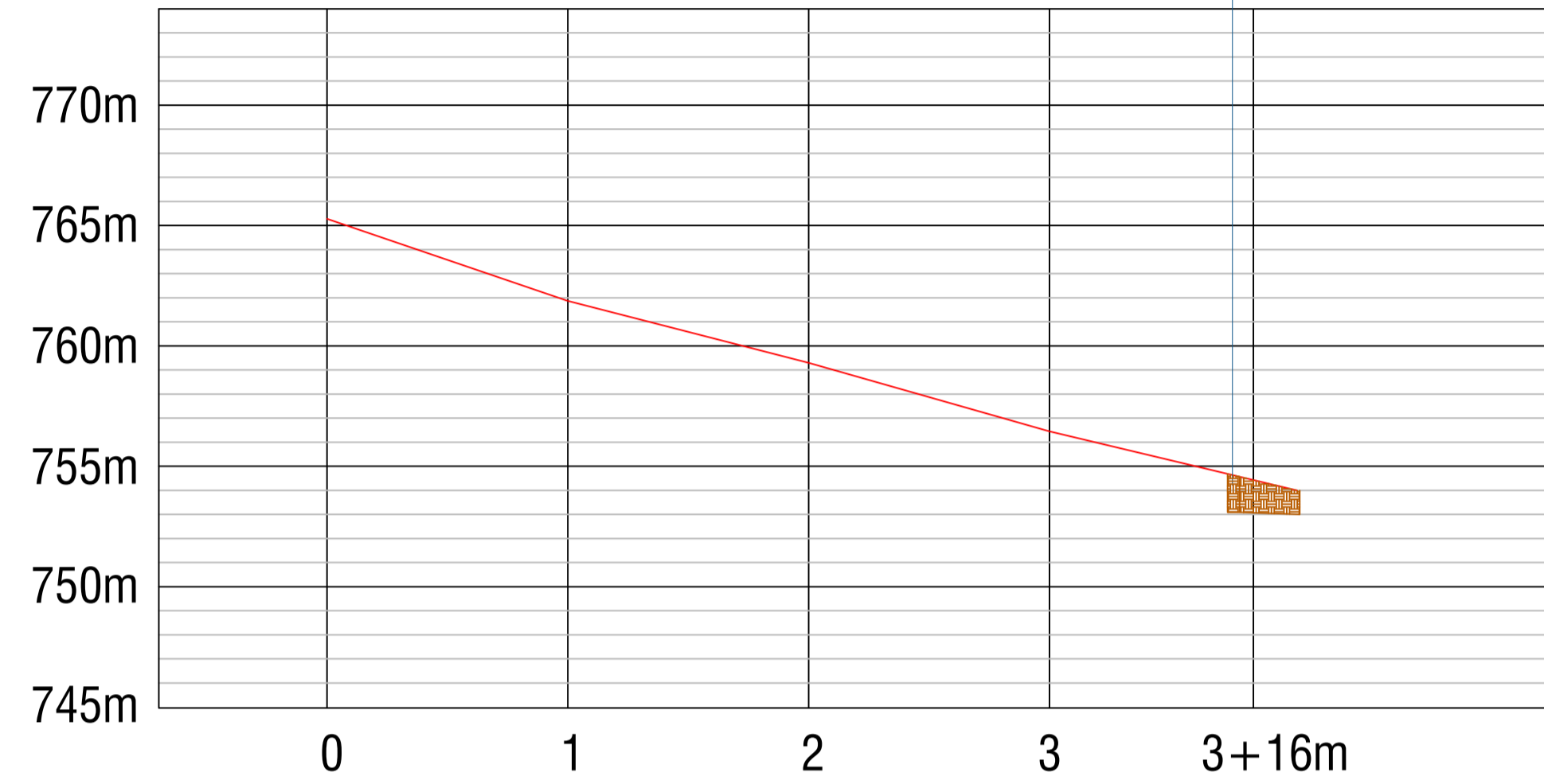
PERFIL LONGITUDINAL - RUA CARLOS FONTANA - Trecho 1 Esc. 1/500
