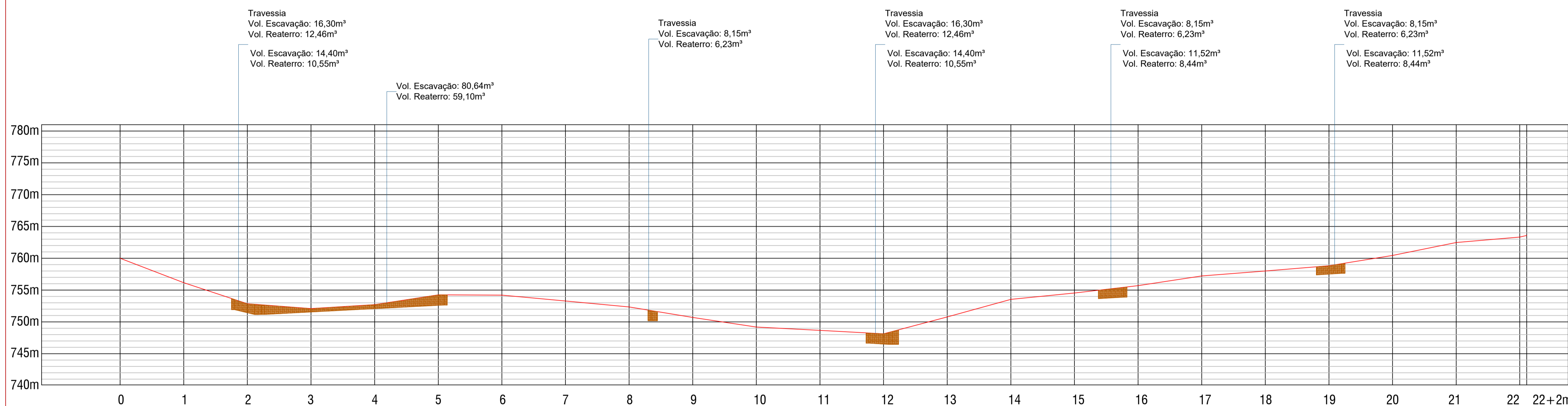
PERFIL LONGITUDINAL - RUA JOSÉ OLDONI Esc. 1/750
