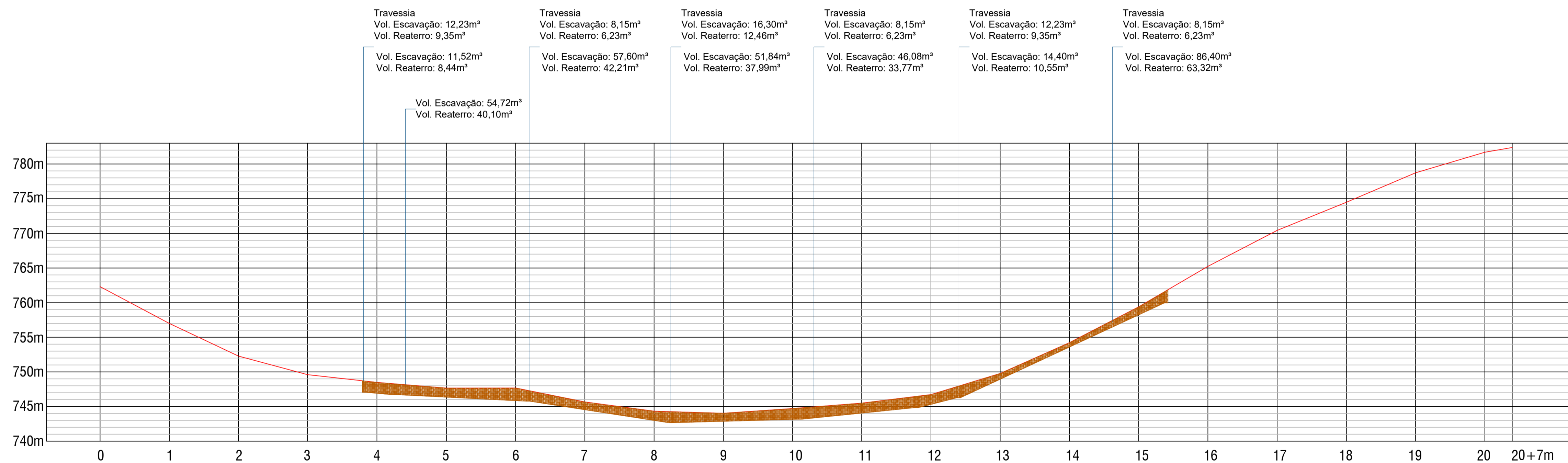
PERFIL LONGITUDINAL - RUA FREDERICO KLEM Esc. 1/750
