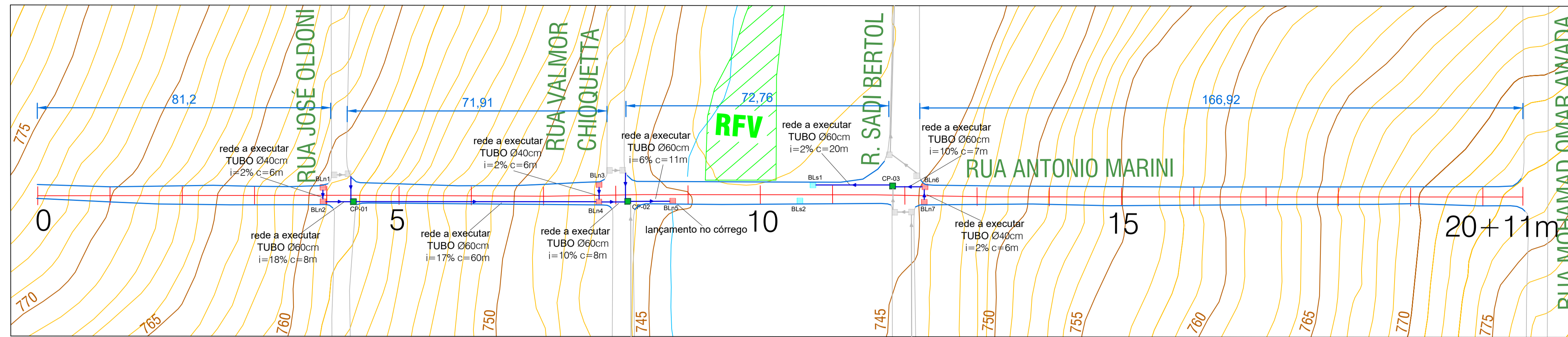
DRENAGEM - RUA ANTÔNIO MARINI Esc. 1/750
