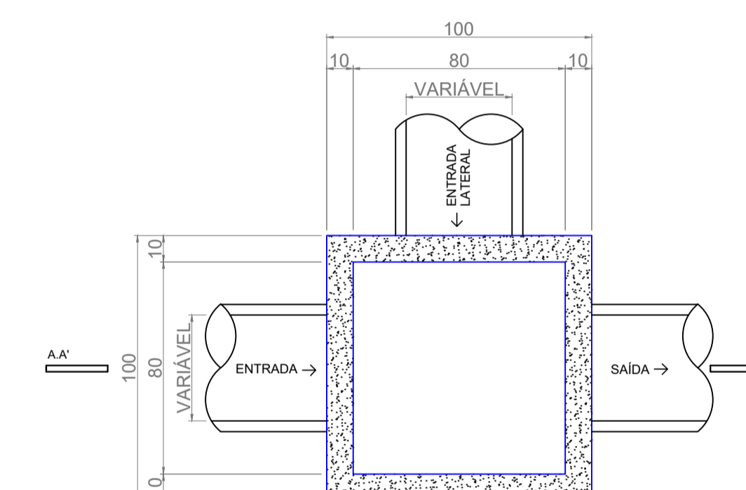
PLANTA BAIXA ESCALA 1/20
