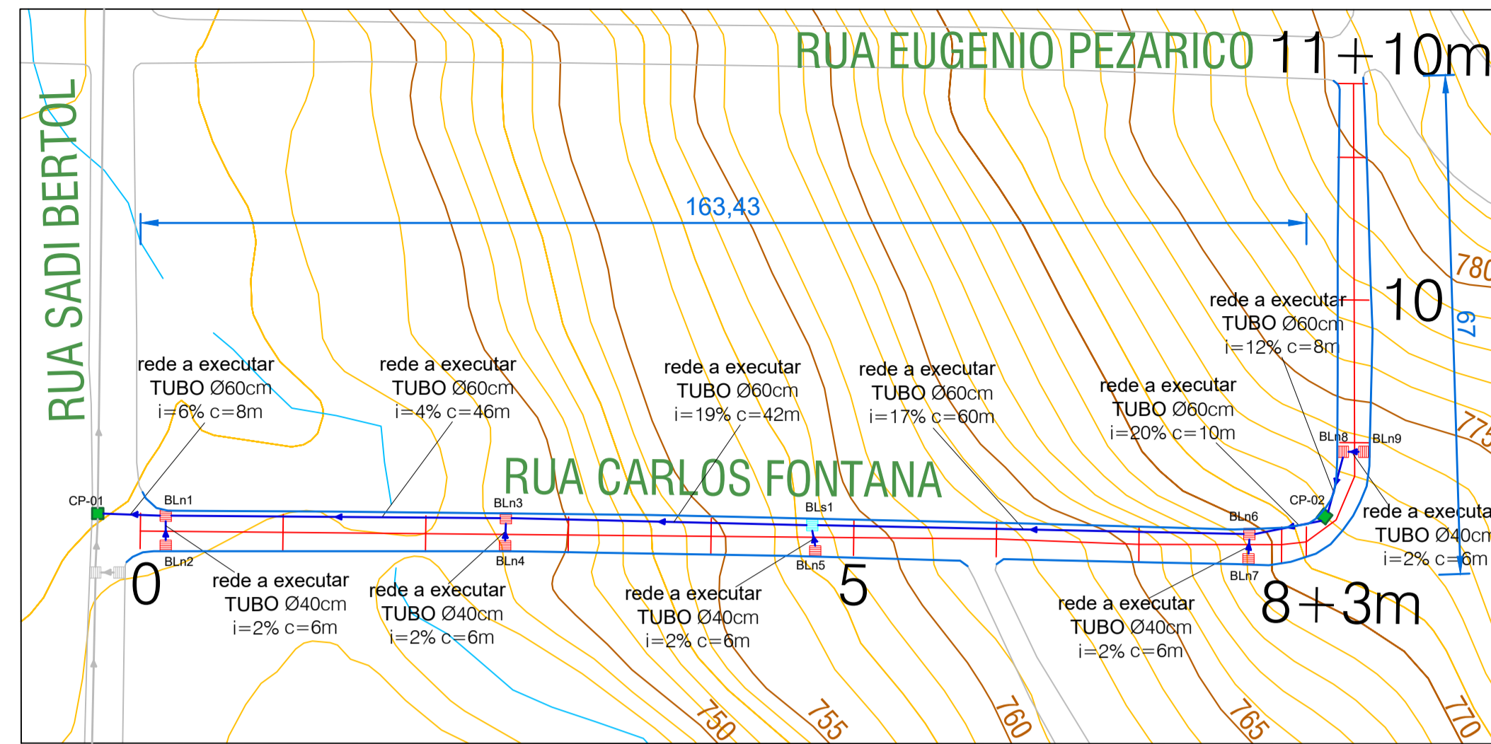
DRENAGEM - RUA CARLOS FONTANA - Trecho 2 Esc. 1/750
