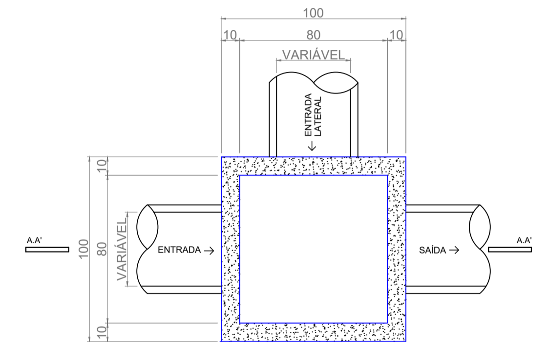
PLANTA BAIXA ESCALA 1/20
