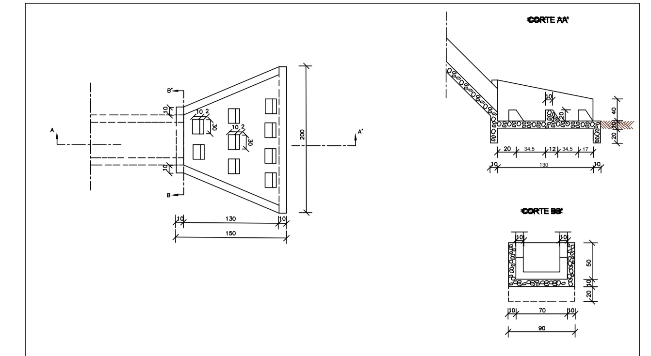
DETALHE DISSIPADOR DE ENERGIA Esc. 1/50
