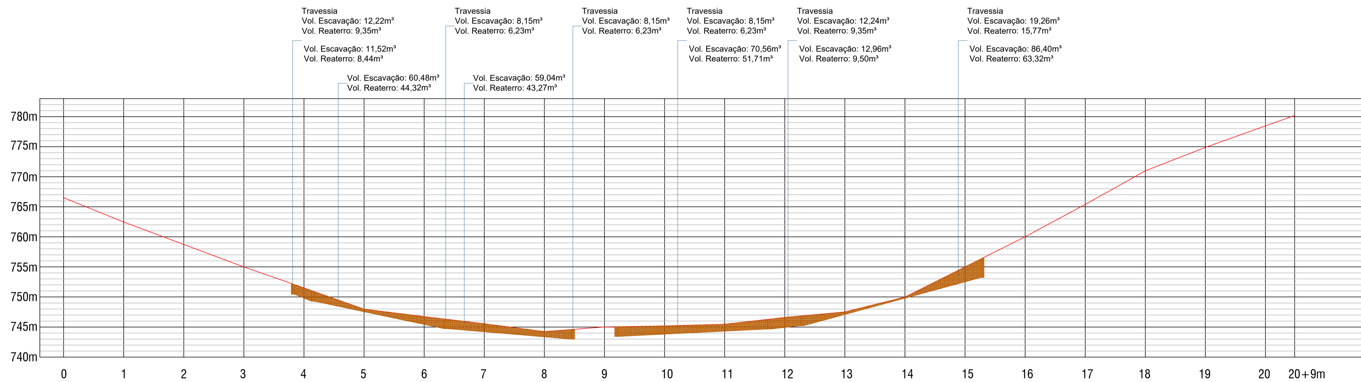
PERFIL LONGITUDINAL - RUA EUGÊNIO PEZARICO Esc. 1/750
