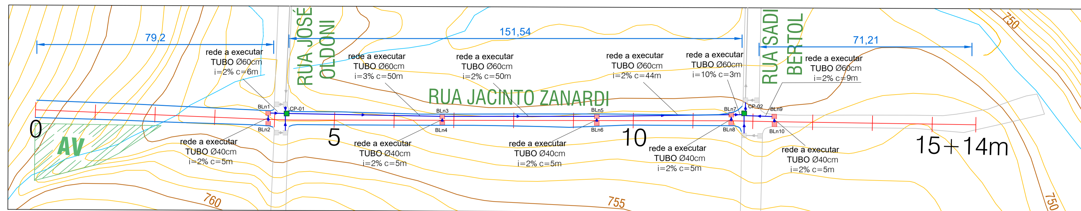
DRENAGEM - RUA JACINTO ZANARDI Esc. 1/750
