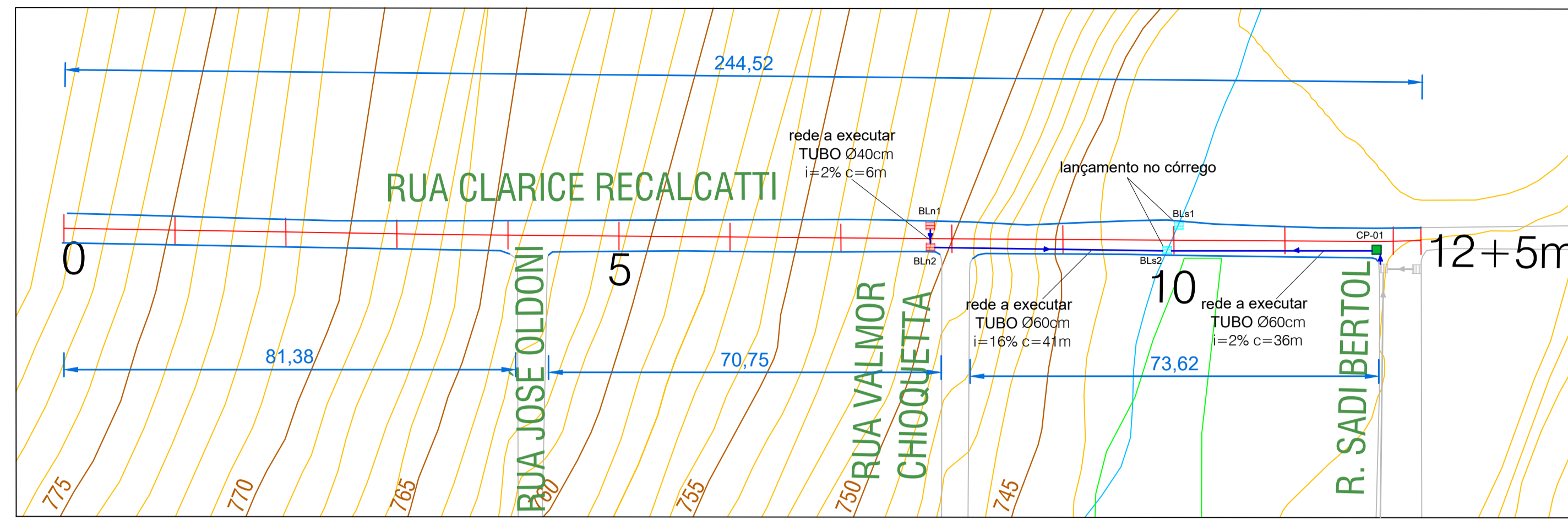
DRENAGEM - RUA CLARICE RECALCATTI Esc. 1/750
