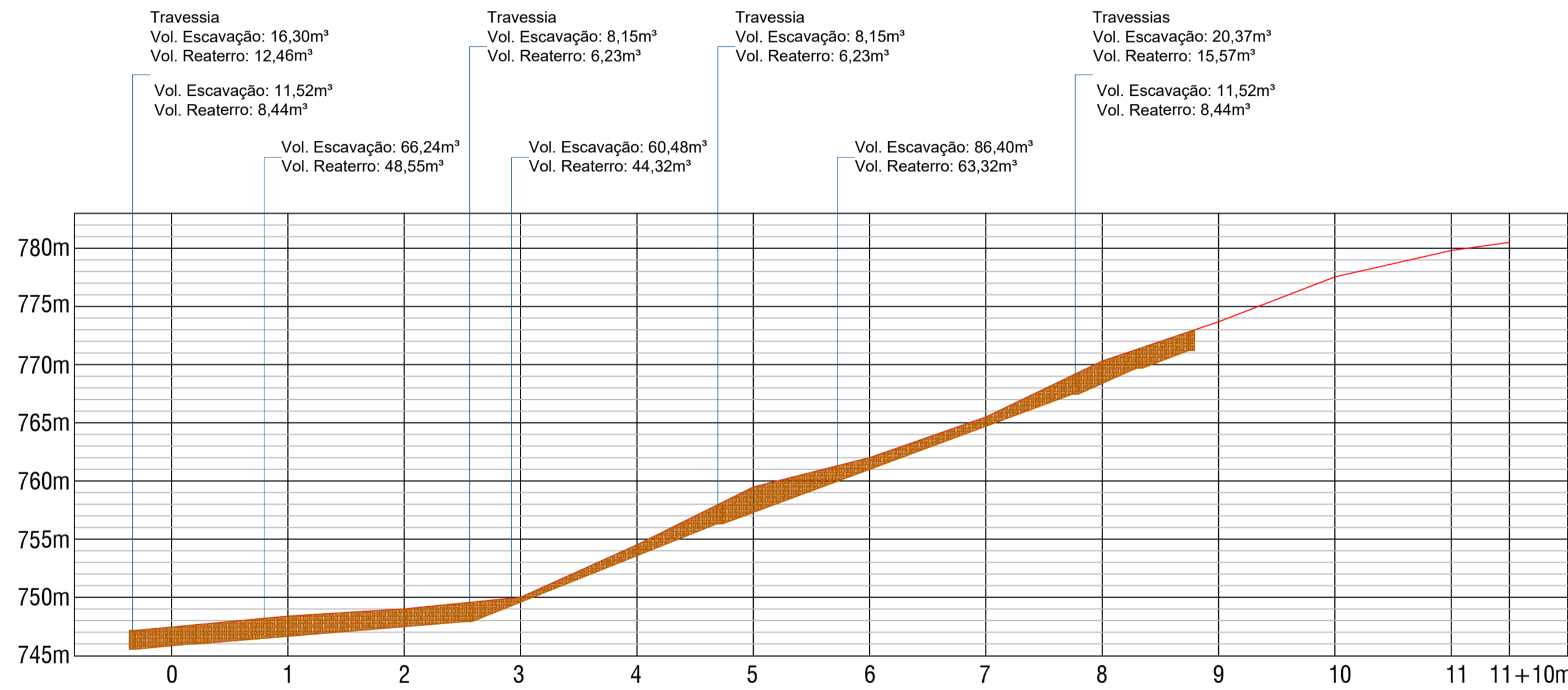
PERFIL LONGITUDINAL - RUA CARLOS FONTANA - Trecho 2 Esc. 1/750
