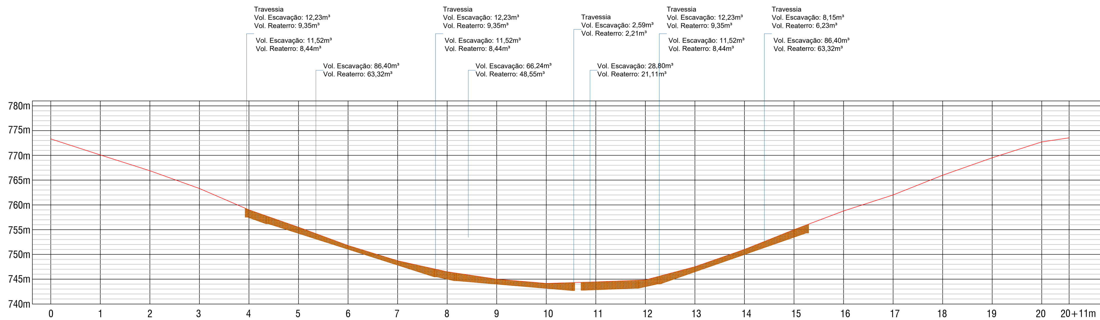
PERFIL LONGITUDINAL - RUA ANTÔNIO MARINI Esc. 1/750
