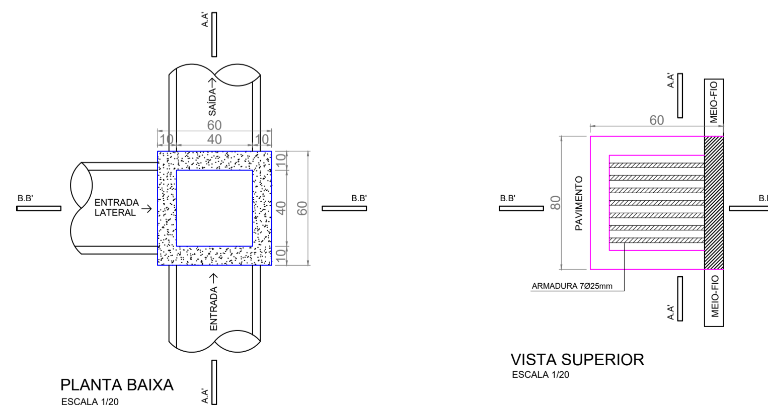
DETALHE BOCA DE LOBO
