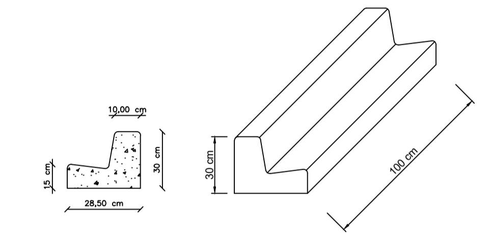
DETALHE MEIO FIO Esc. 1/20
