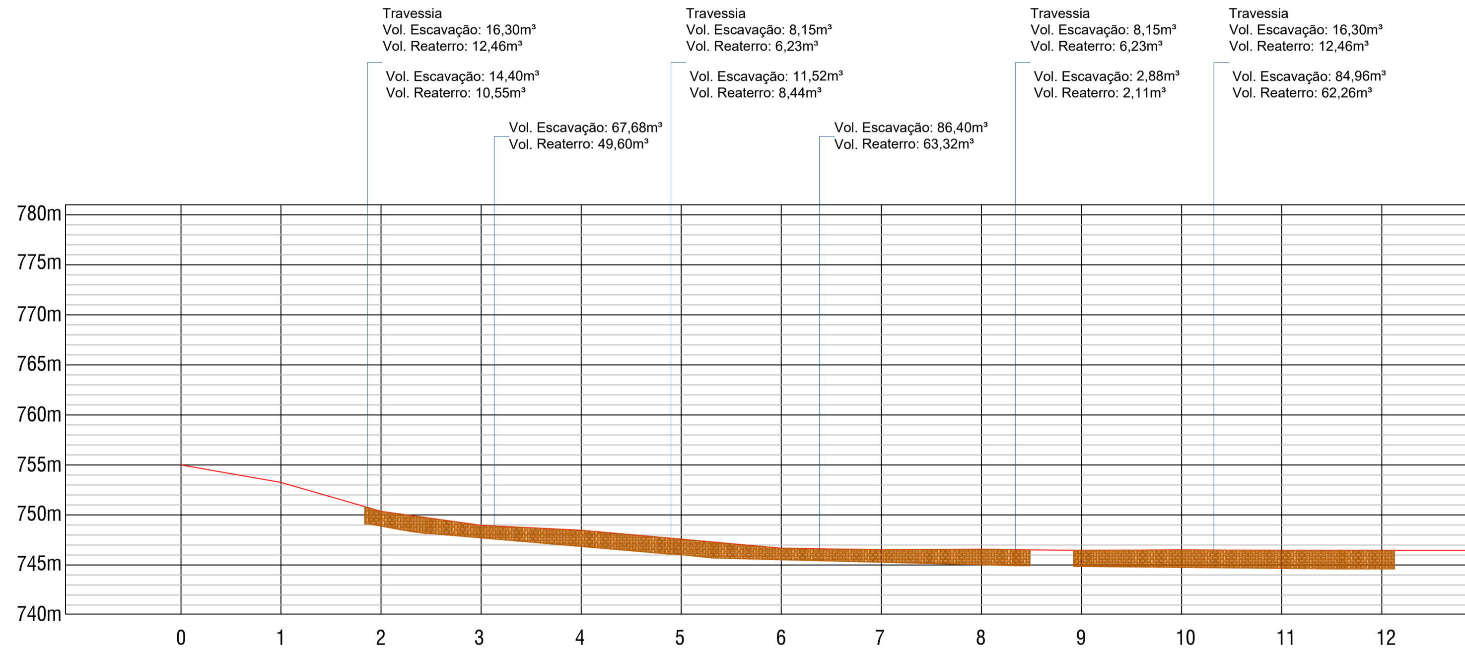
PERFIL LONGITUDINAL - RUA SADI BERTOL Esc. 1/750
