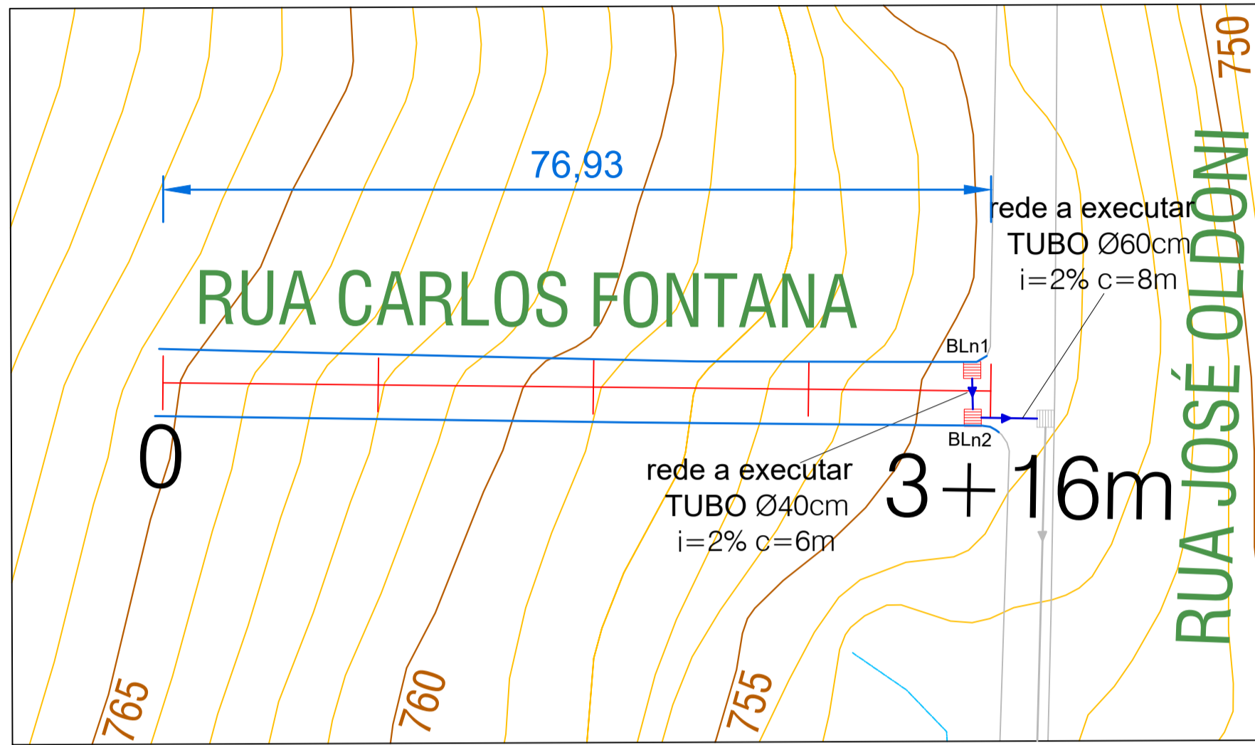
DRENAGEM - RUA CARLOS FONTANA - Trecho 1 Esc. 1/500
