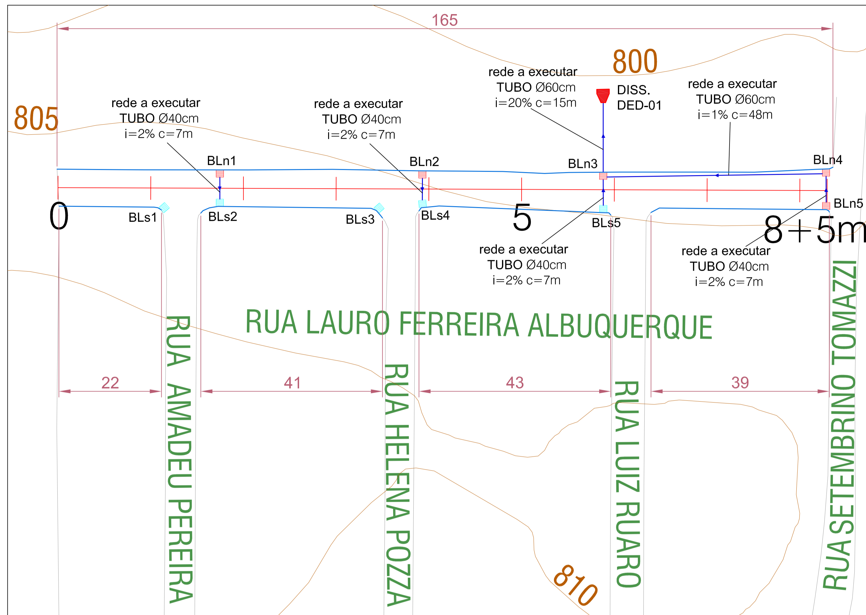
DRENAGEM E MEIO FIO - RUA LAURO FERREIRA ALBUQUERQUE Esc. 1/500
