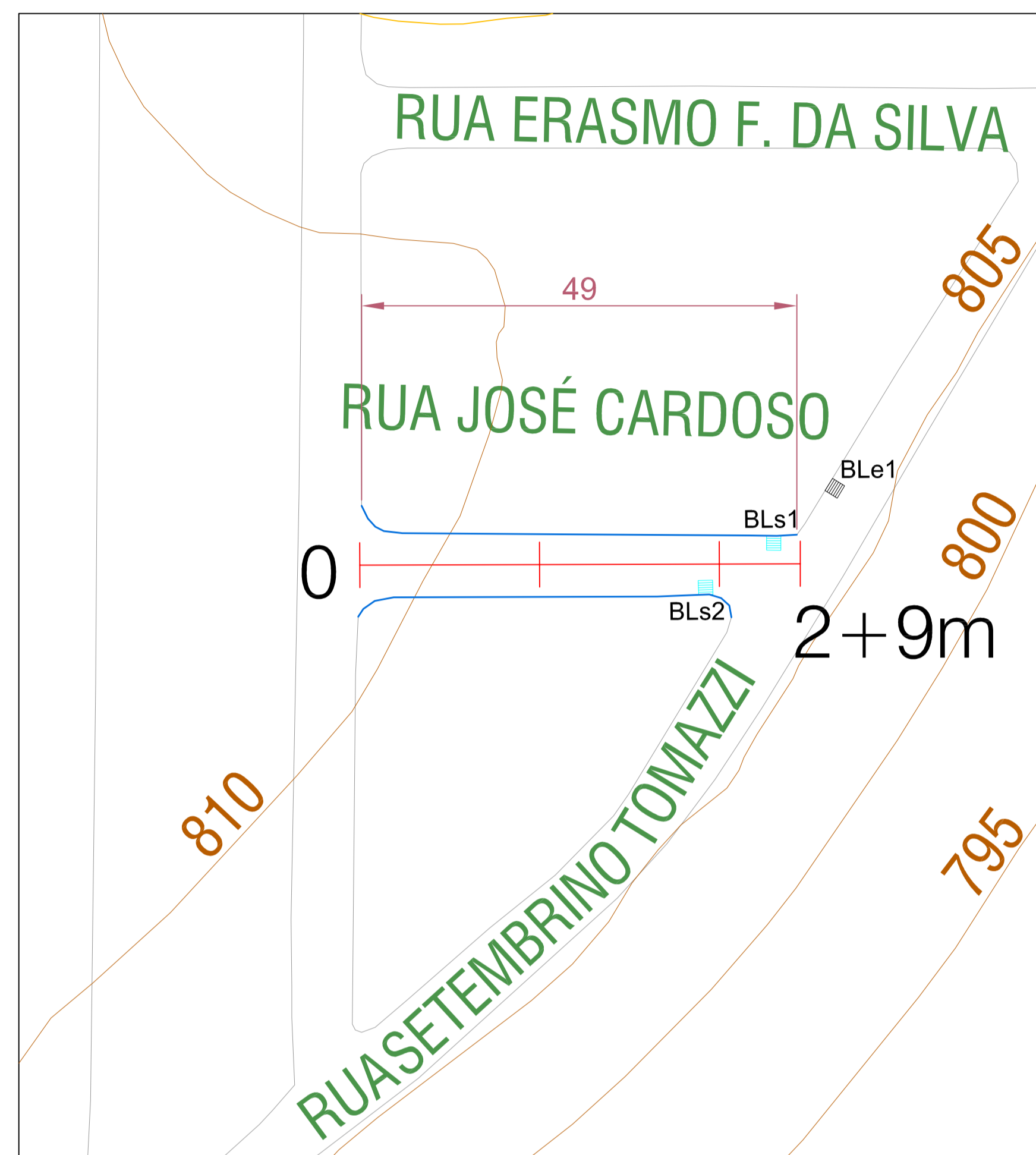
DRENAGEM E MEIO FIO - RUA JOSÉ CARDOSO Esc. 1/500
