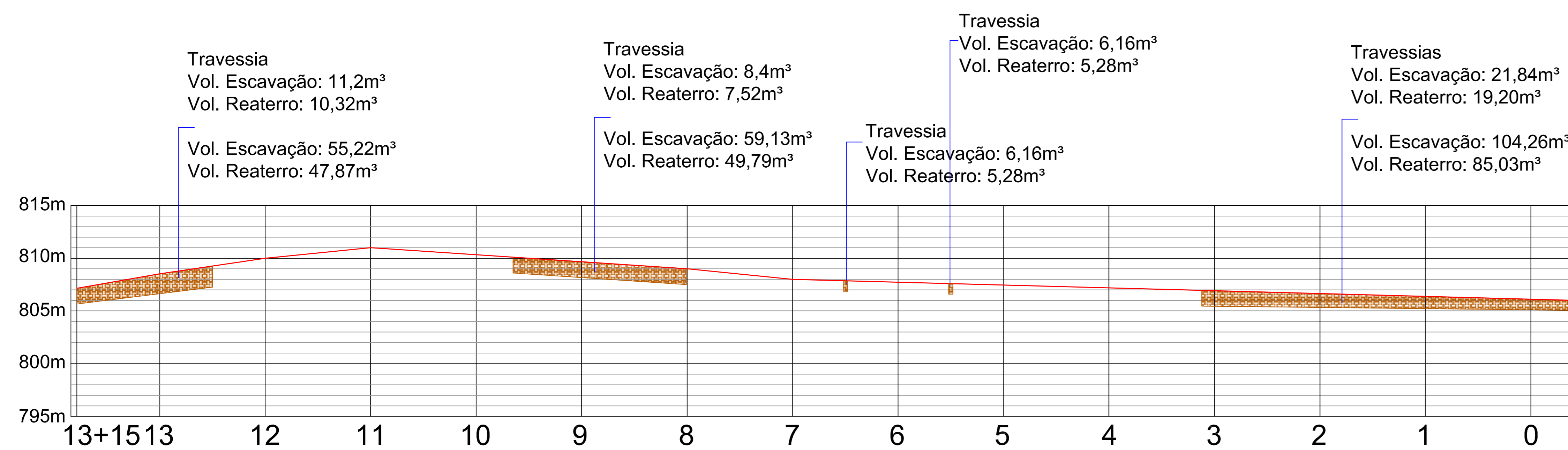
PERFIL LONGITUDINAL - RUA AMADEU PEREIRA Esc. 1/500
