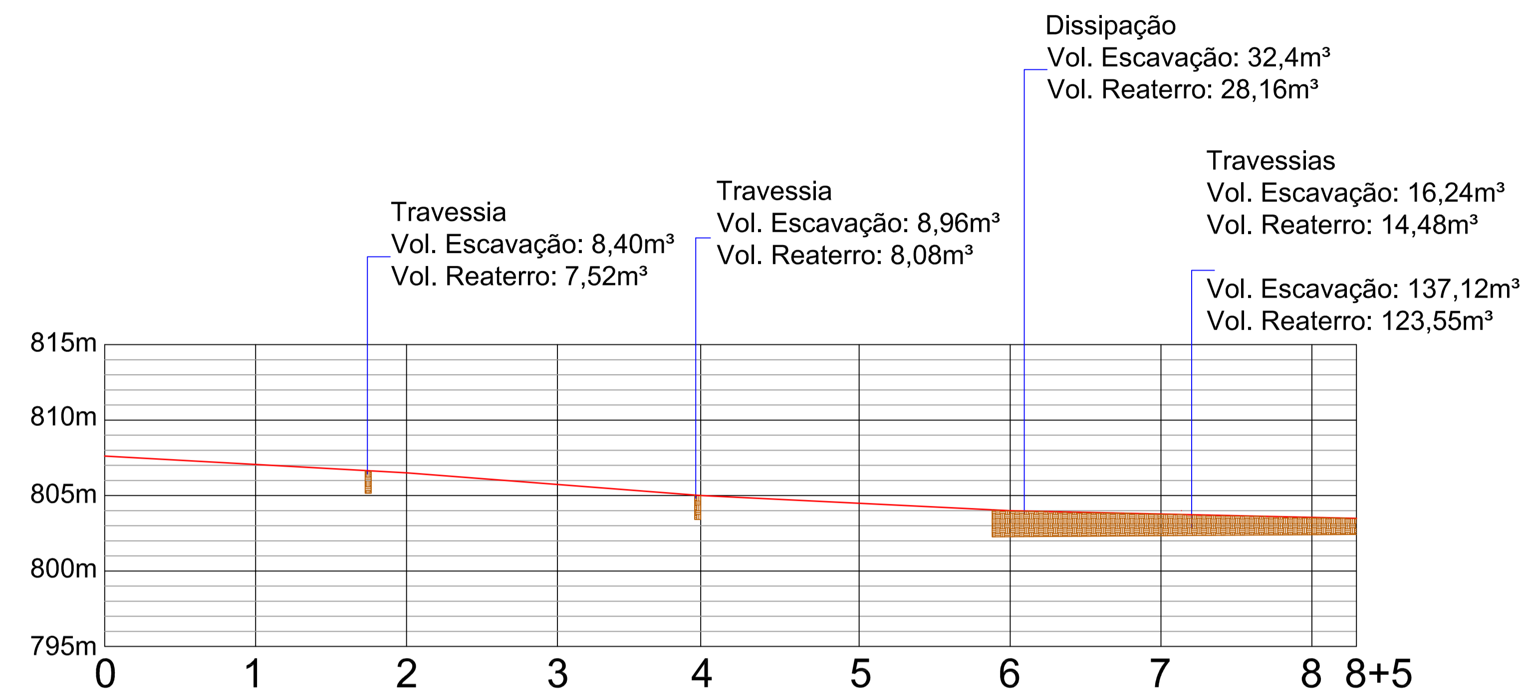
PERFIL LONGITUDINAL - RUA LAURO FERREIRA ALBUQUERQUE Esc. 1/500
