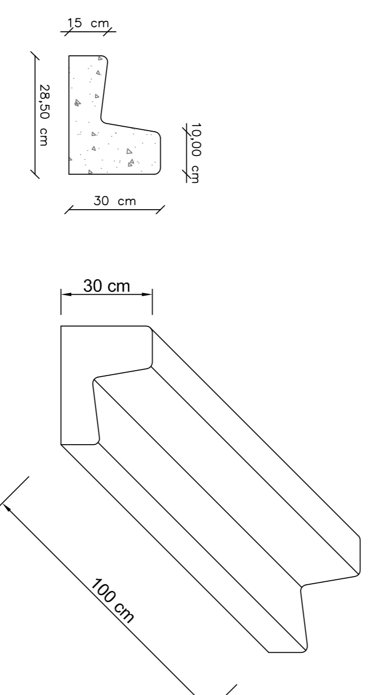
DETALHE MEIO FIO SEM ESCALA
