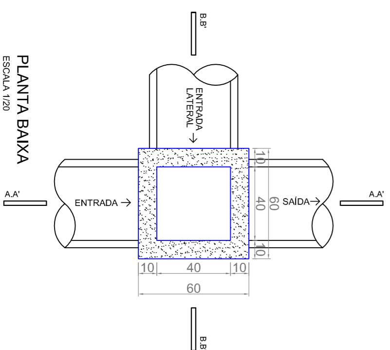
BOCA DE LOBO
