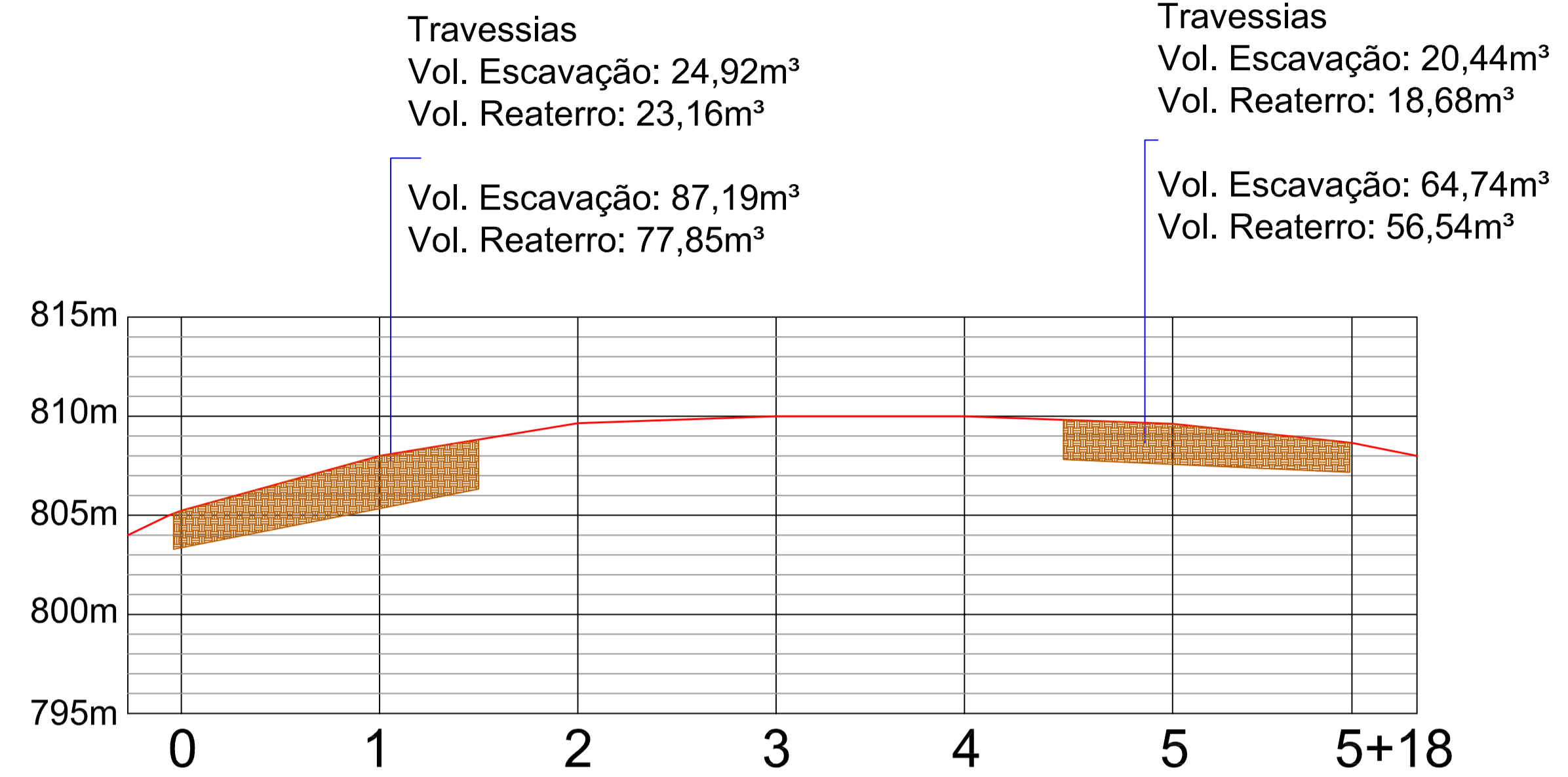
PERFIL LONGITUDINAL - RUA LUIZ RUARO Esc. 1/500
