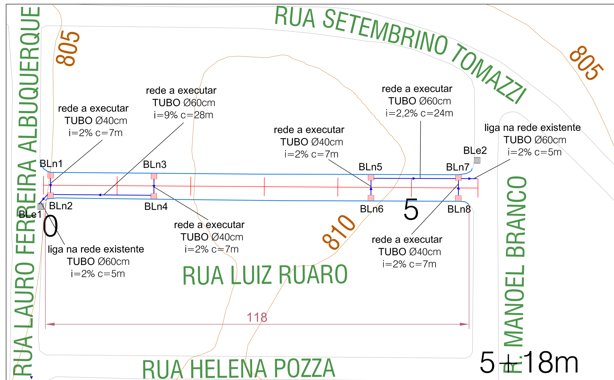
DRENAGEM E MEIO FIO - RUA LUIZ RUARO Esc. 1/500
