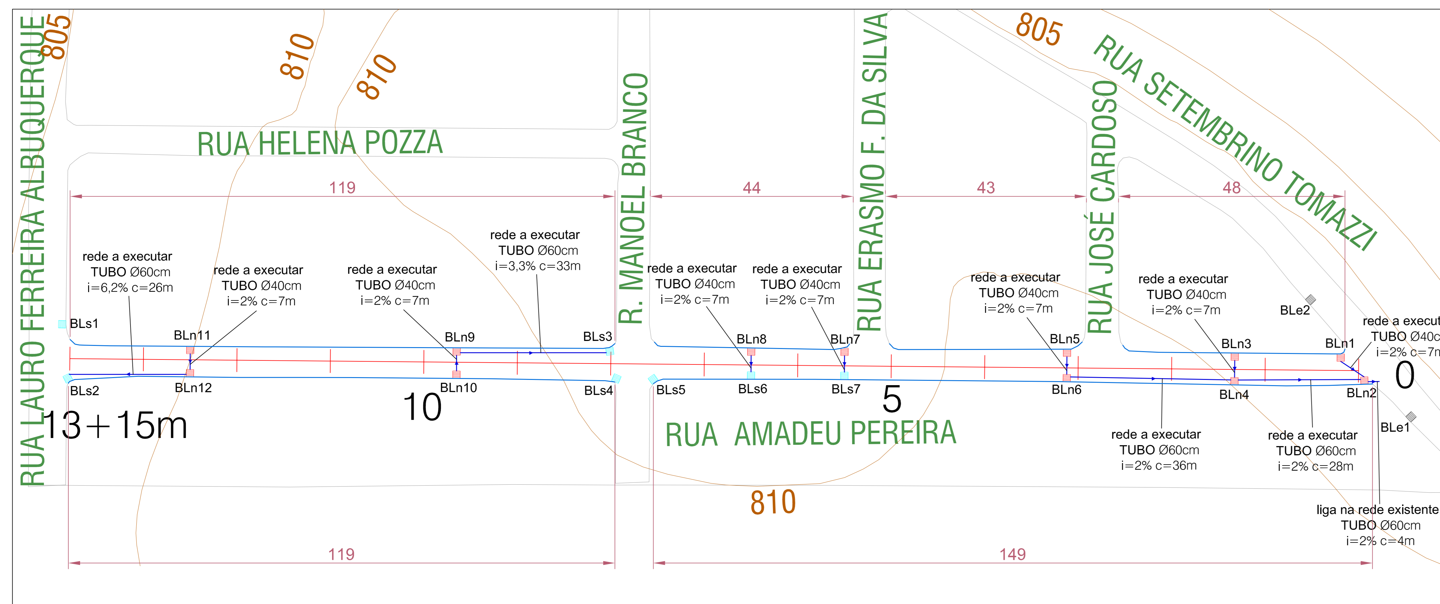
DRENAGEM E MEIO FIO - RUA AMADEU PEREIRA Esc. 1/500
