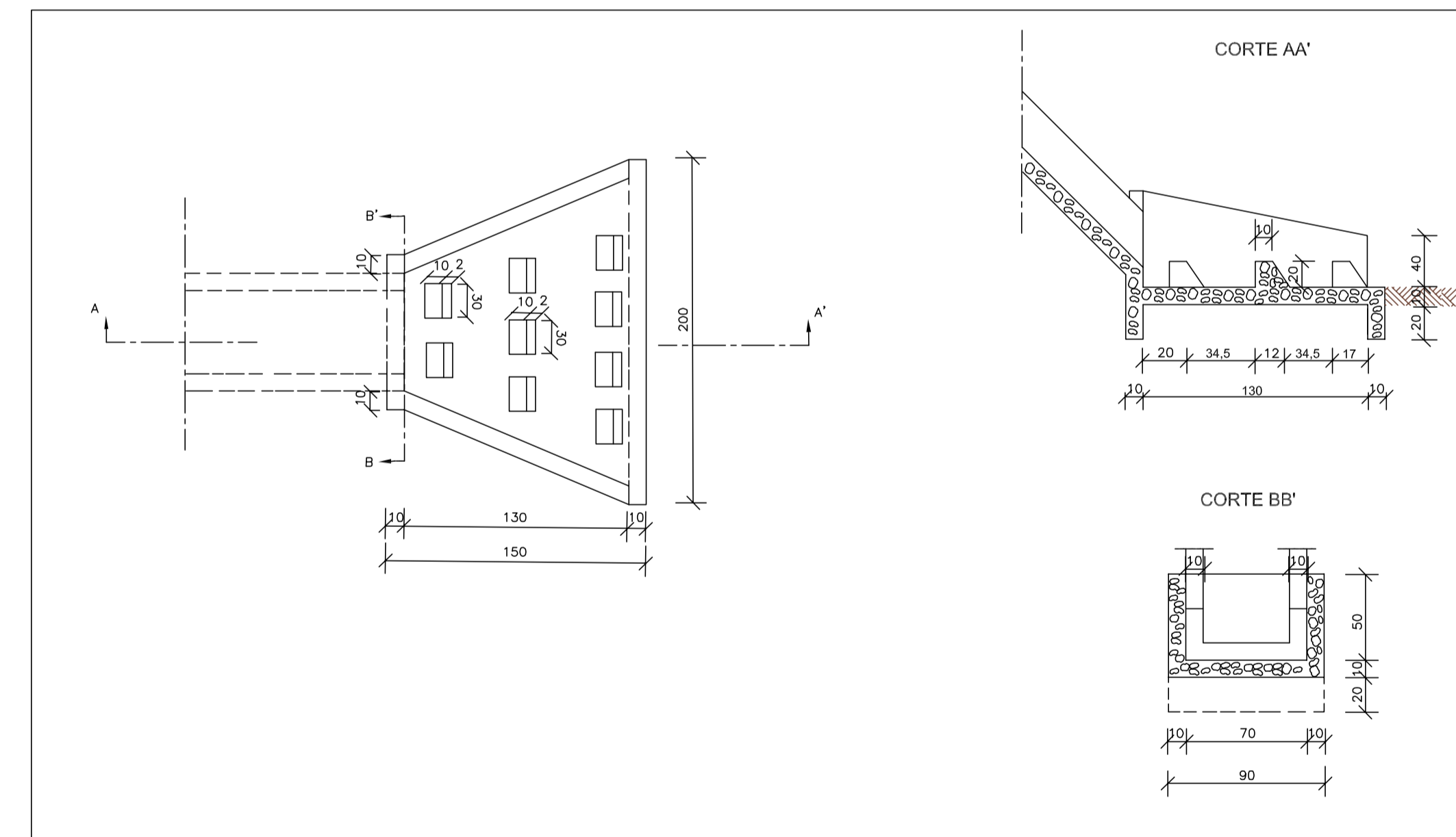
DETALHE DISSIPADOR DE ENERGIA Esc. 1/50
