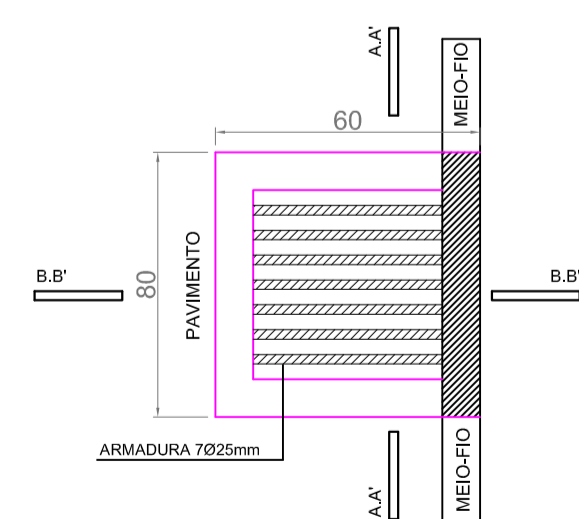
VISTA SUPERIOR ESCALA 1/20
