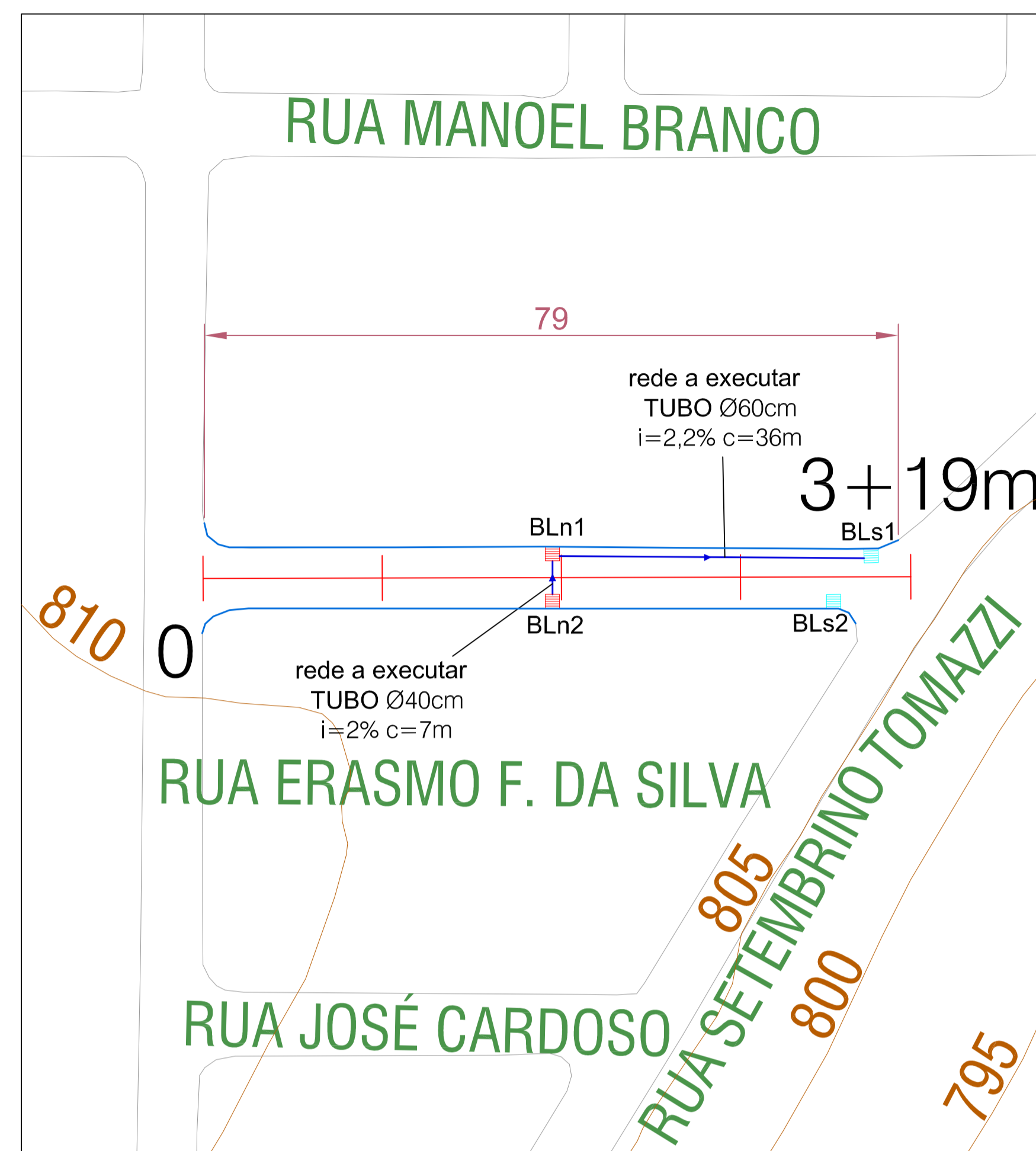
DRENAGEM E MEIO FIO - RUA ERASMO F. DA SILVA Esc. 1/500
