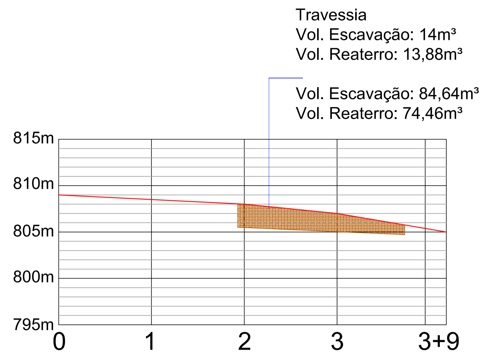
PERFIL LONGITUDINAL - RUA ERASMO F. DA SILVA Esc. 1/500
