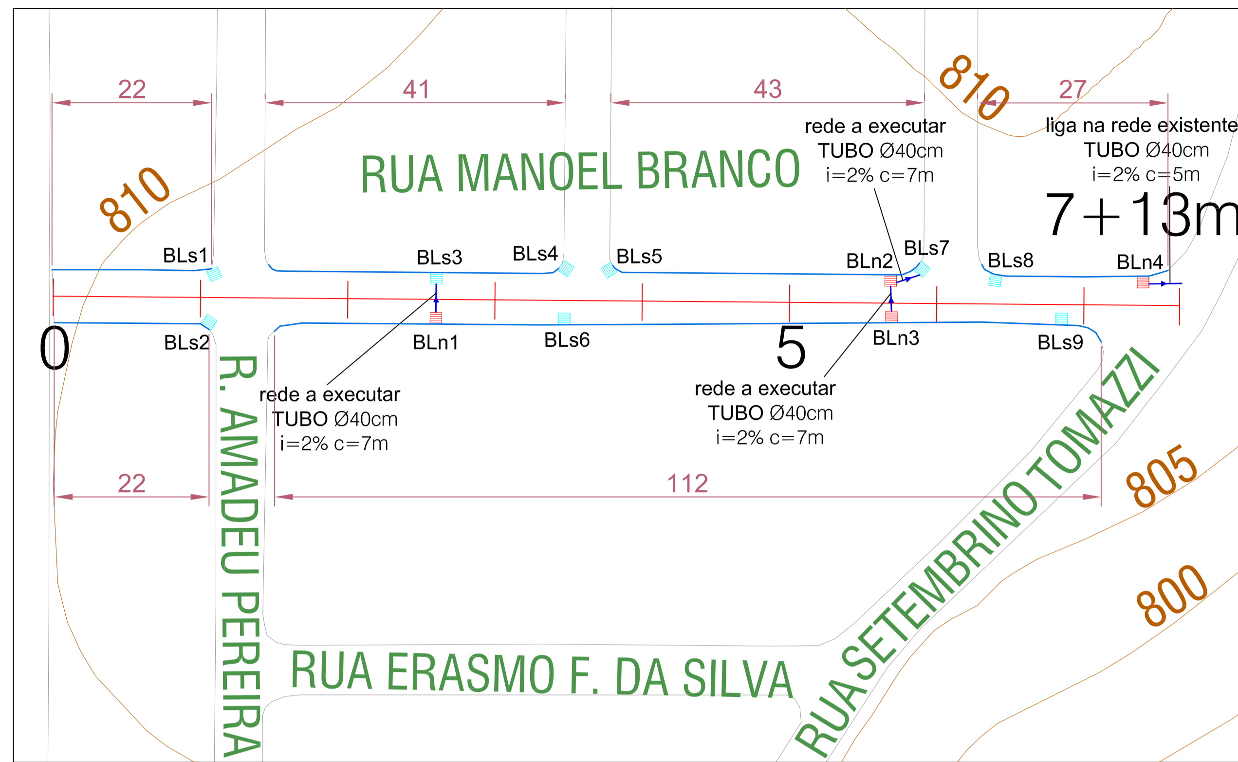
DRENAGEM E MEIO FIO - RUA MANOEL BRANCO Esc. 1/500
