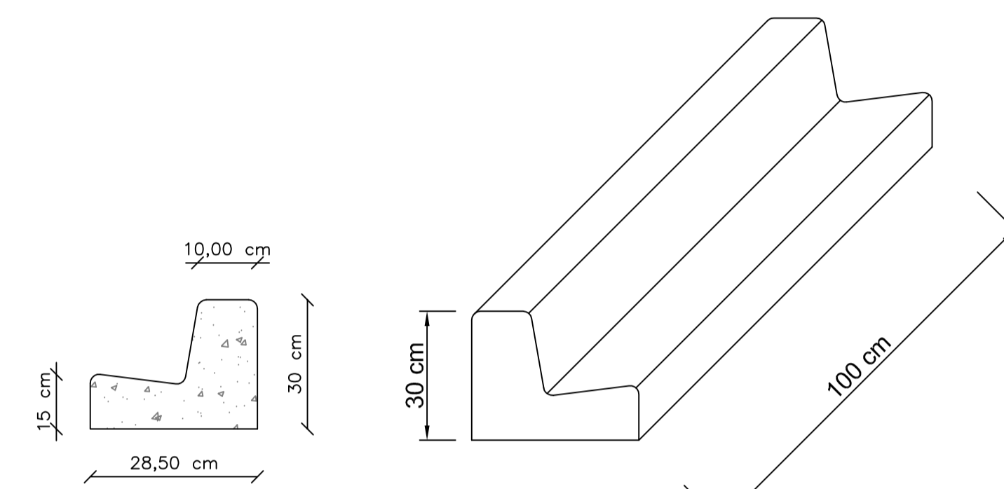
DETALHE MEIO FIO SEM ESCALA
