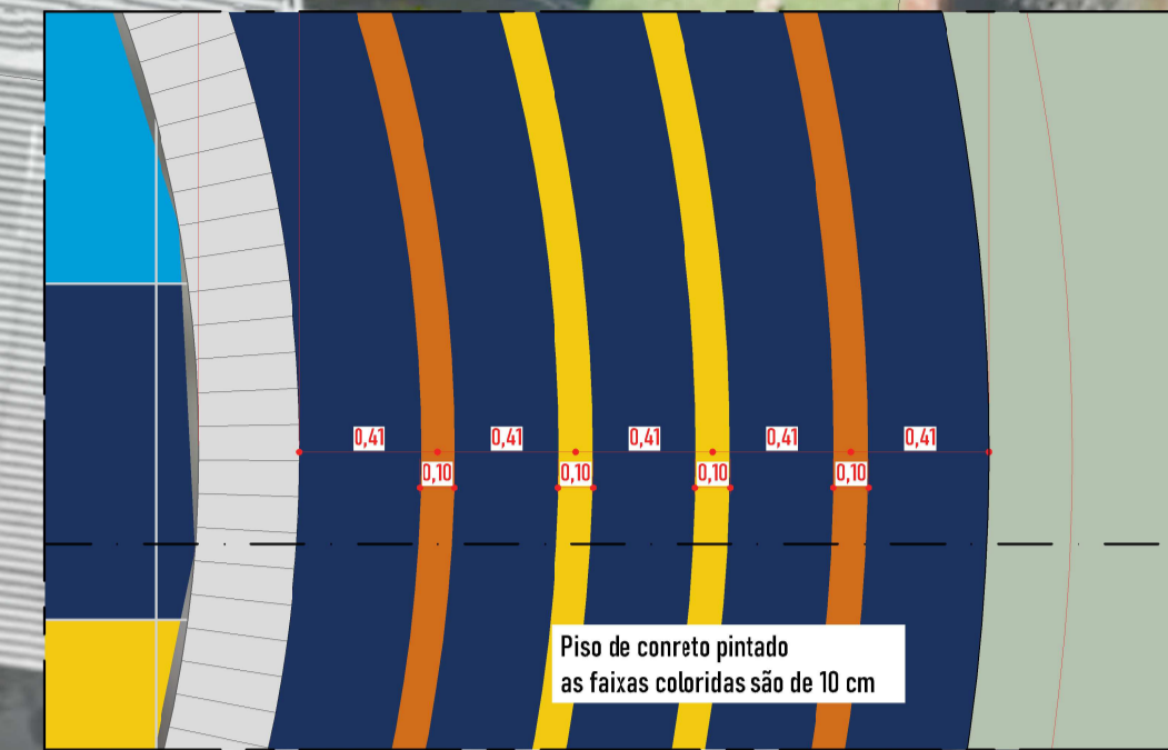
DETALHE PISTA DE CAMINHADA ESC:1/25
