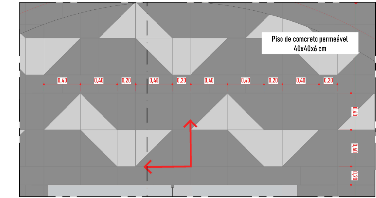
DETALHE DE PISO 02 ESC:1/25
