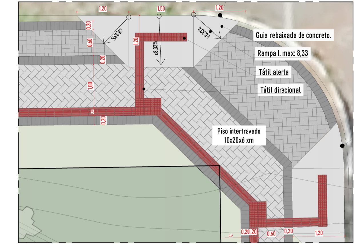
DETALHE DE PISO 03 ESC:1/50
