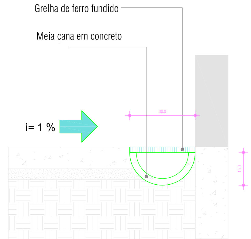
1 - Detalhe Canaleta S/ESC
