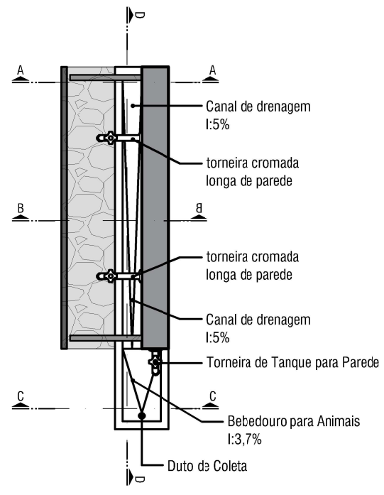
PLANTA BAIXA ESC: 1/20
