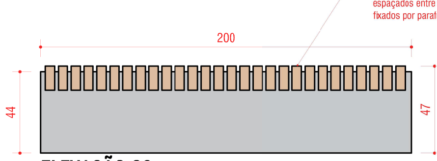
ELEVAÇÃO 02 ESC: 1/20
