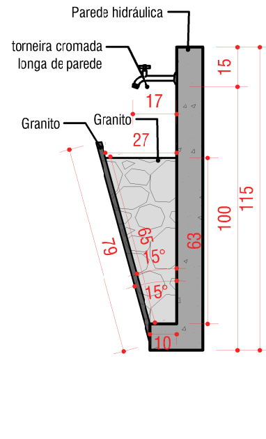
CORTE A ESC: 1/20
