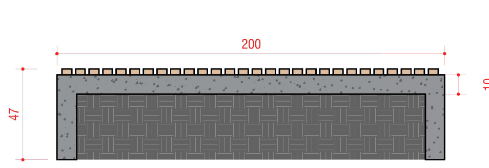
CORTE A ESC: 1/20
