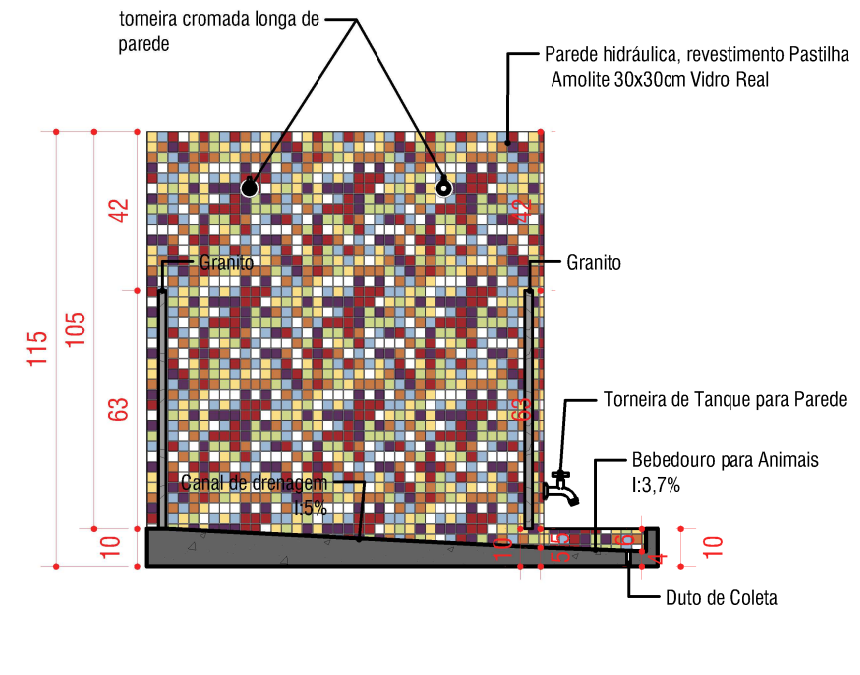
CORTE D ESC: 1/20
