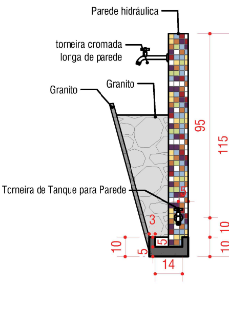
CORTE C ESC: 1/20
