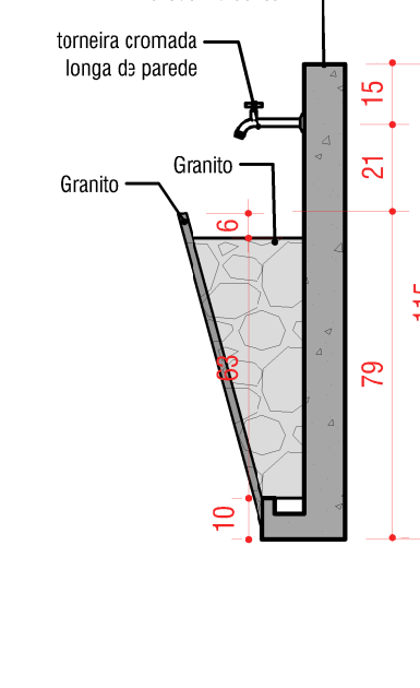
CORTE B ESC: 1/20
