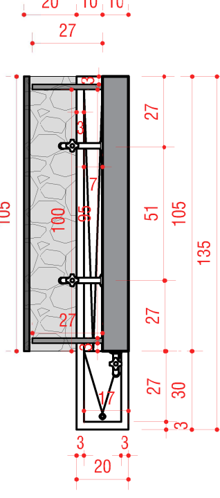
PLANTA BAIXA ESC: 1/20
