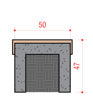
CORTE B ESC: 1/20
