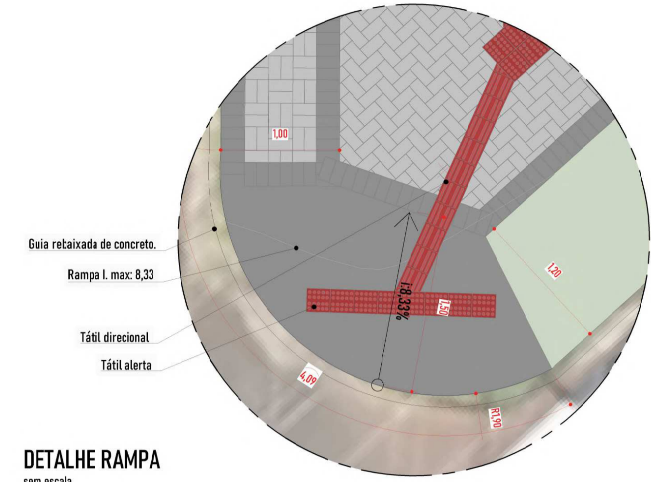
DETALHE DO PISO sem escala
