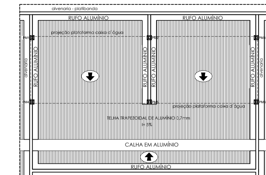
03 PLANTA DE COBERTURA SOB CAIXAS D'ÁGUA ESQ. 1:10
