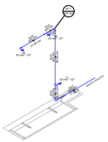
ISOMÉTRICO ESCALA 1:25
