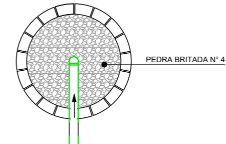
PLANTA BAIXA - SUMIDOURO SEM ESCALA
