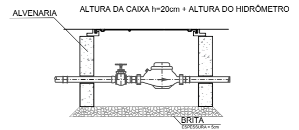
CORTE CAIXA SEM ESCALA
