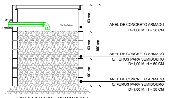
VISTA LATERAL - SUMIDOURO SEM ESCALA
