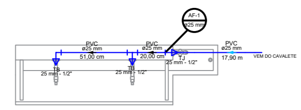
PLANTA BAIXA ESCALA 1:25
