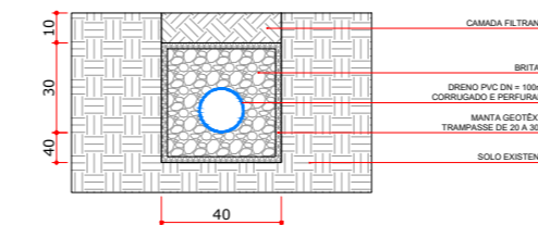
DETALHE DRENO SUBSUPERFICIAL SEM ESCALA
