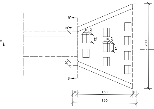
PLANTA BAIXA
