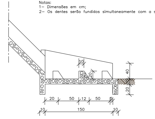
CORTE AA'
