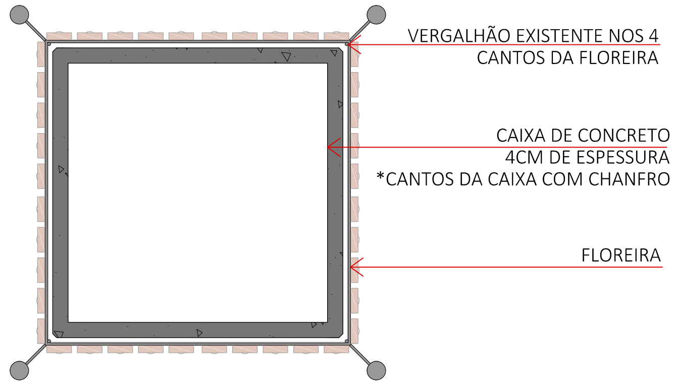
VISTA SUPERIOR - FLOREIRA + CAIXA DE CONCRETO ESC: 1/10
