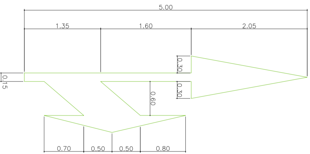
DETALHE 02 S/ESCALA
