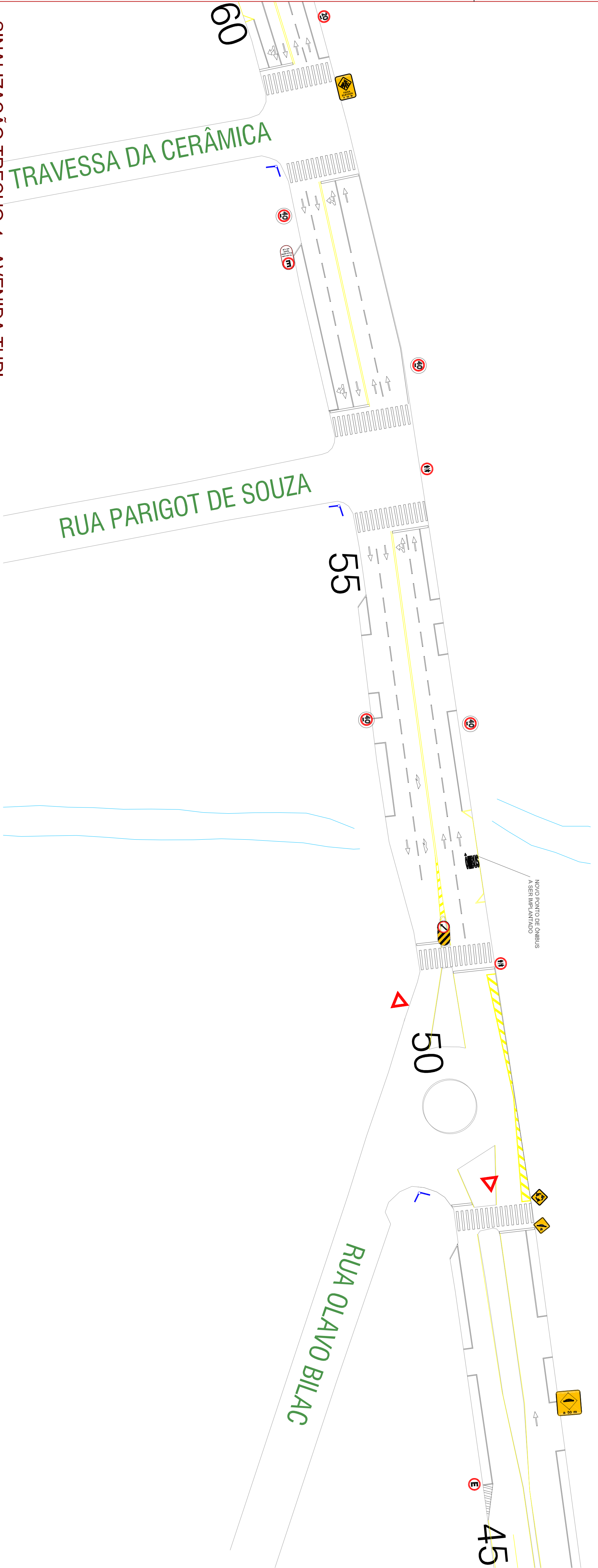
SINALIZAÇÃO TRECHO 3- AVENIDA TUPI ESCALA 1:500
