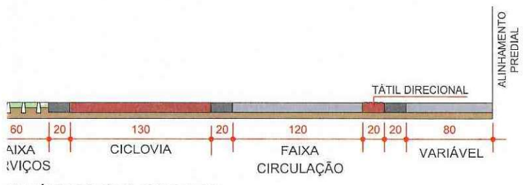
EMÁTICO CALÇADA 5B
