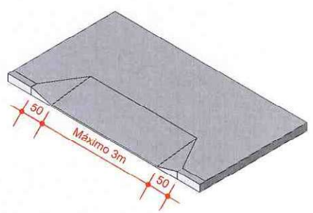
DET. GUIA REBAIXADA PARA VEÍCULOS
