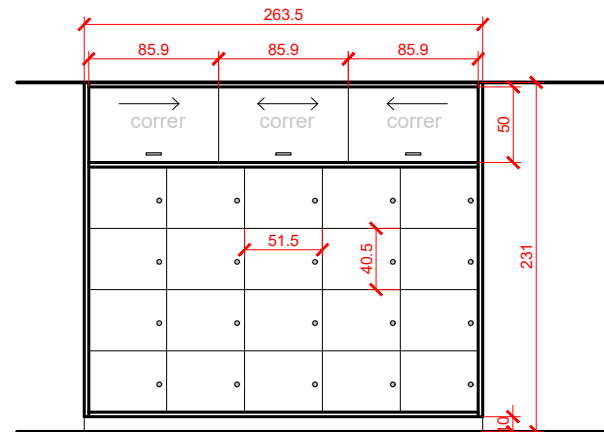
VISTA 01 ESC: 1/50
