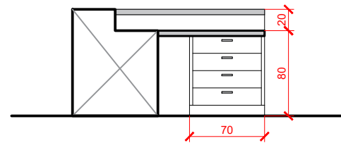
VISTA 01 ESC: 1/50
