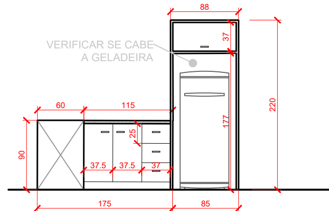
VISTA 02 ESC: 1/50
