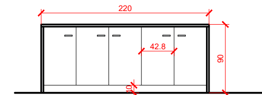
VISTA 01 ESC: 1/50
