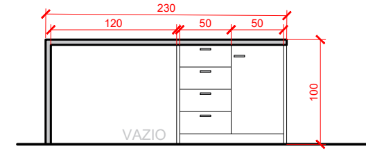
VISTA 01 ESC: 1/50
