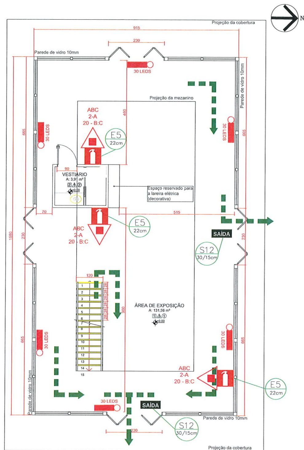
PLANTA BAIXA PAVIMENTO INFERIOR Escala: 1/50 Área: 131,56m²
