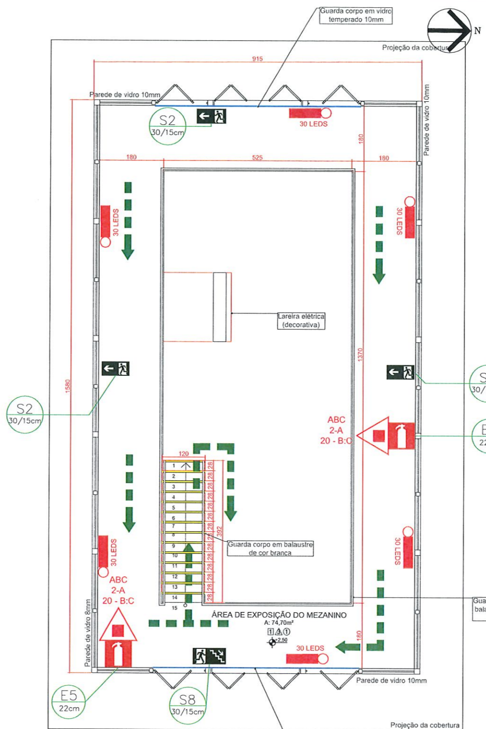
PLANTA BAIXA PAVIMENTO DO MEZANINO Escala: 1/50 Área: 74,70m²
