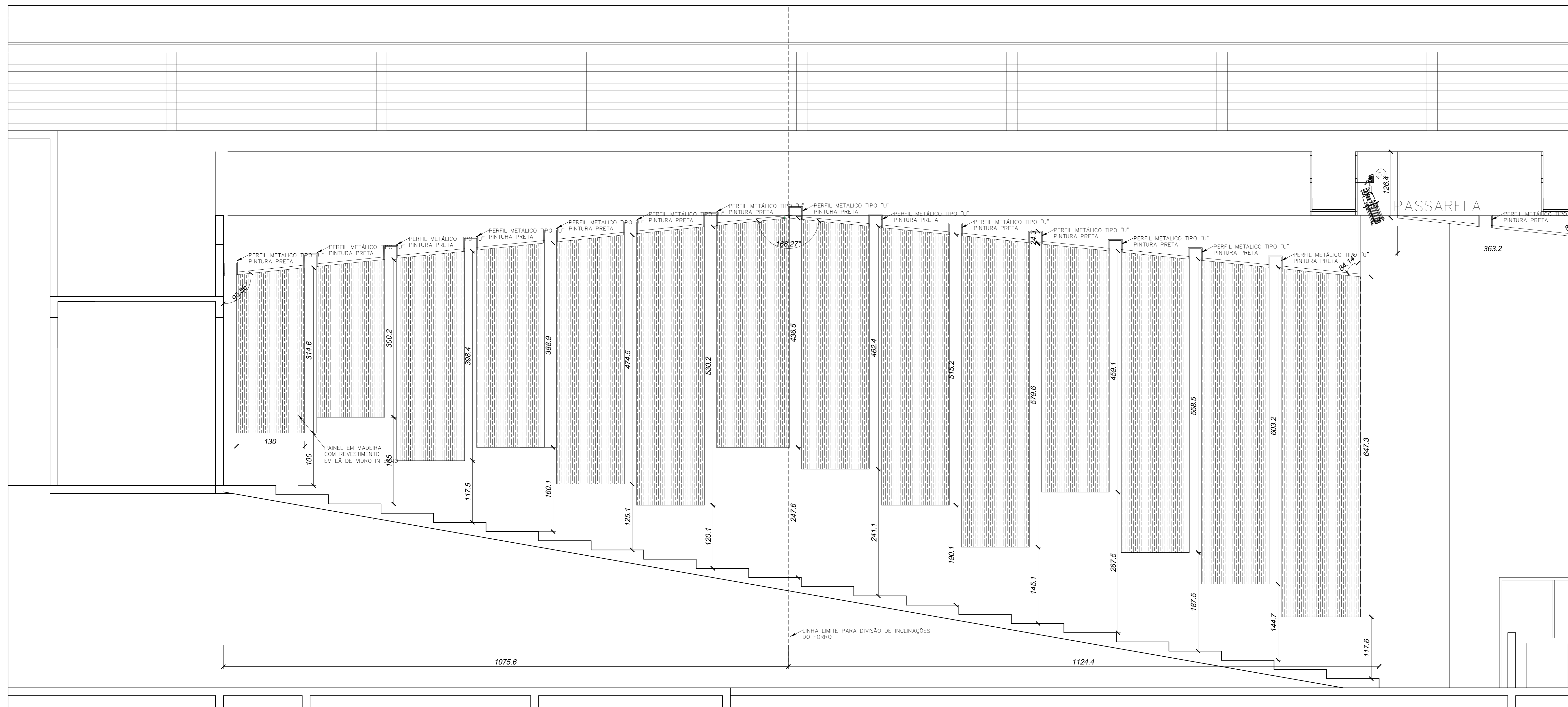
VISTA ANFITEATRO - Layout revestimento de revestimento acústico nas paredes ESCALA 1/50
