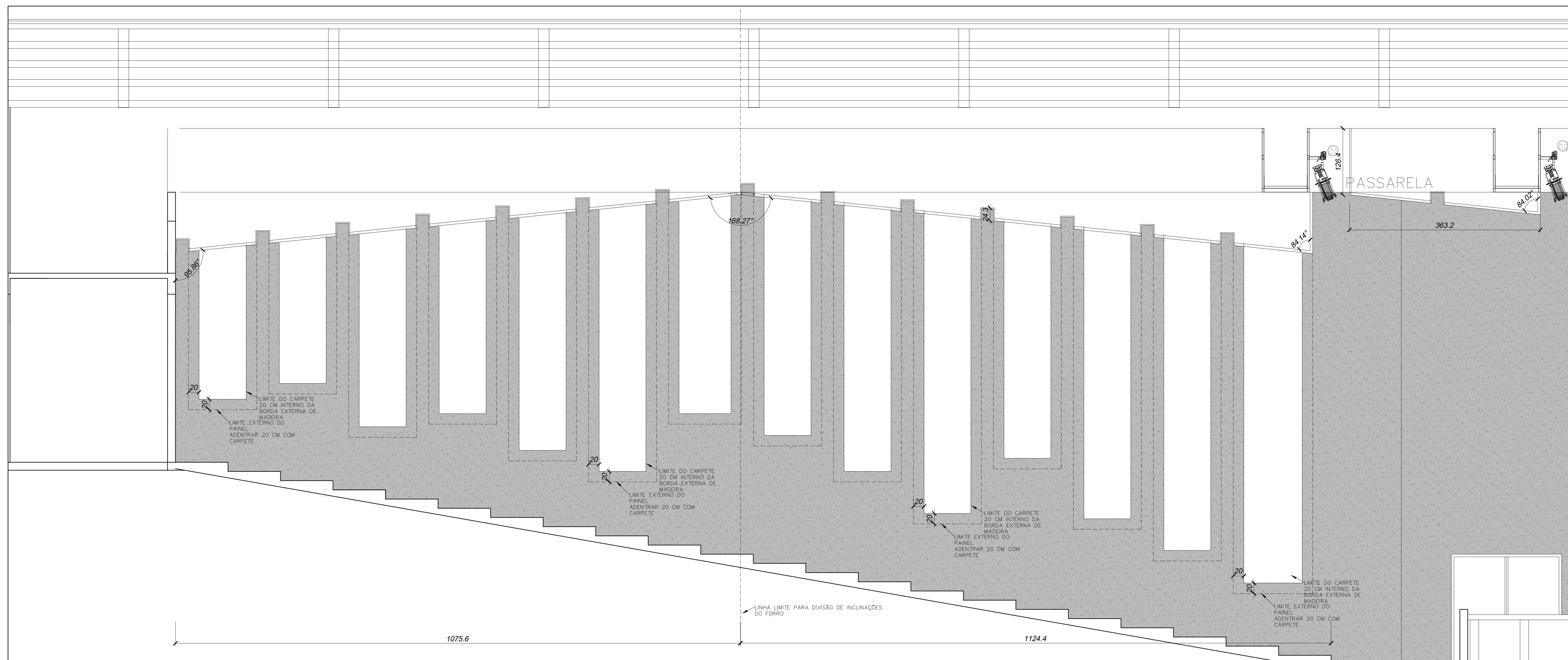
VISTA ANFITEATRO - Layout revestimento de carpete nas paredes ESCALA 1/50
