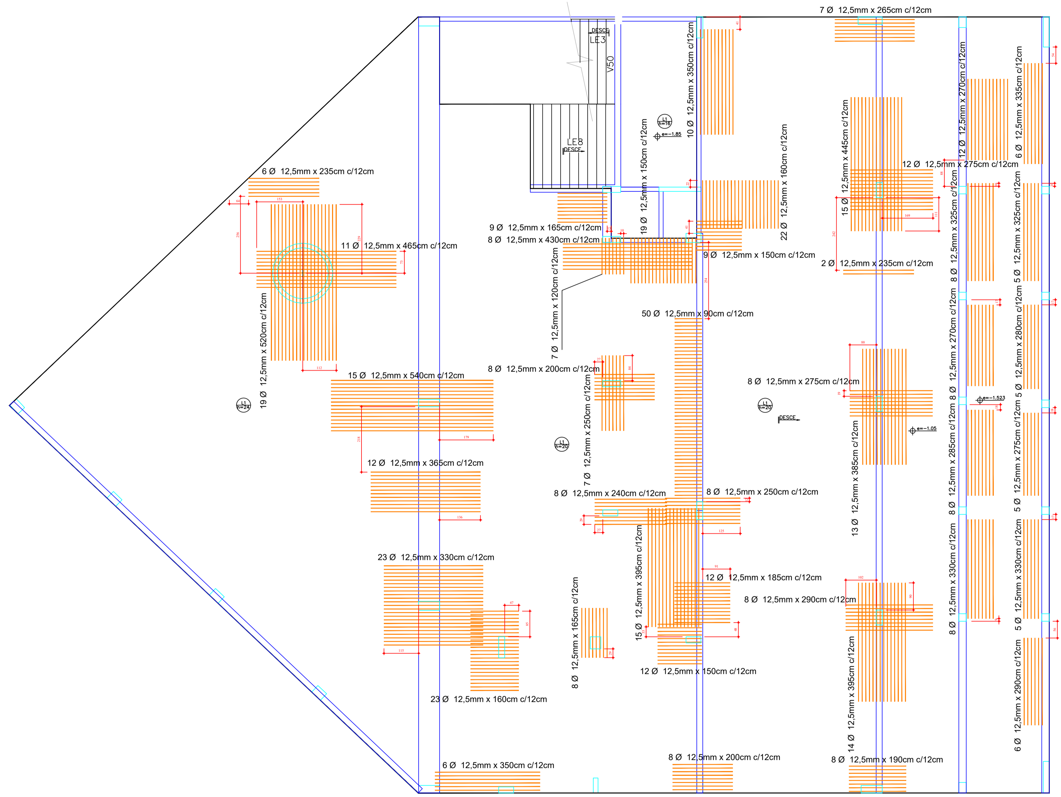
ARMADURA NEGATIVA Esc: 1:75
