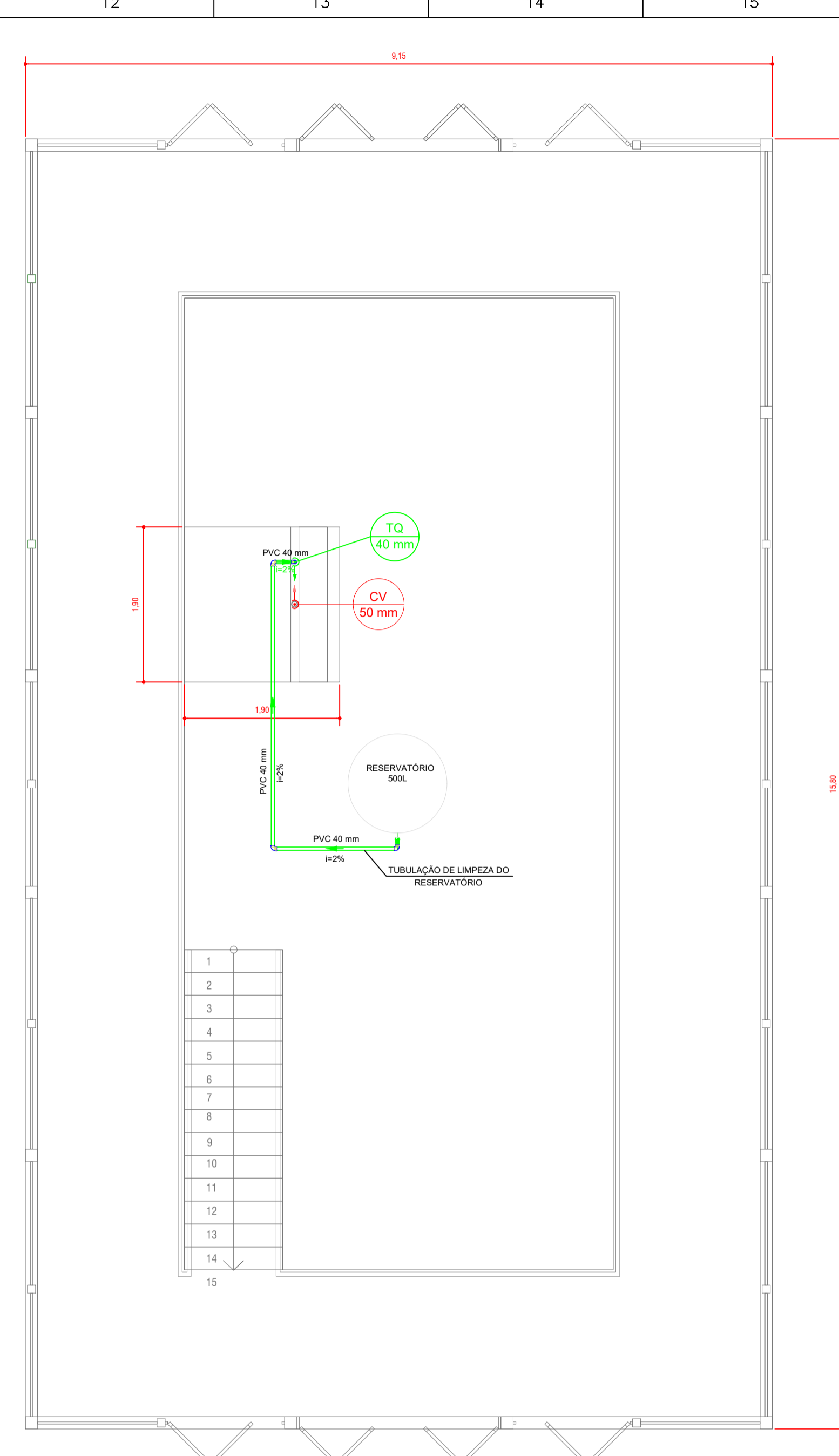
PLANTA BAIXA DO PROJETO DE ESGOTO COBERTURA Escala 1:100
