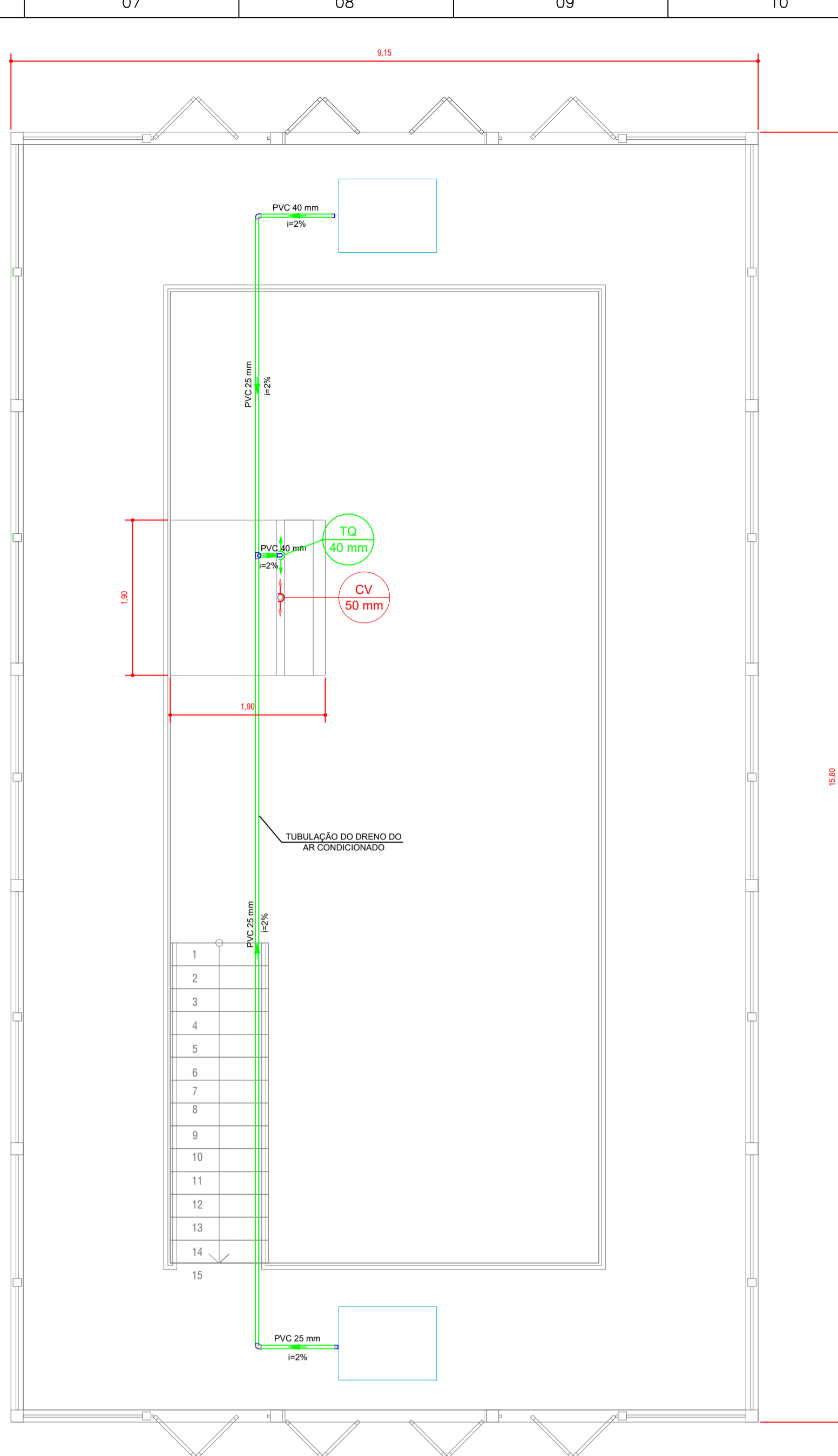
PLANTA BAIXA DO PROJETO DE ESGOTO PAVIMENTO SUPERIOR Escala 1:100
