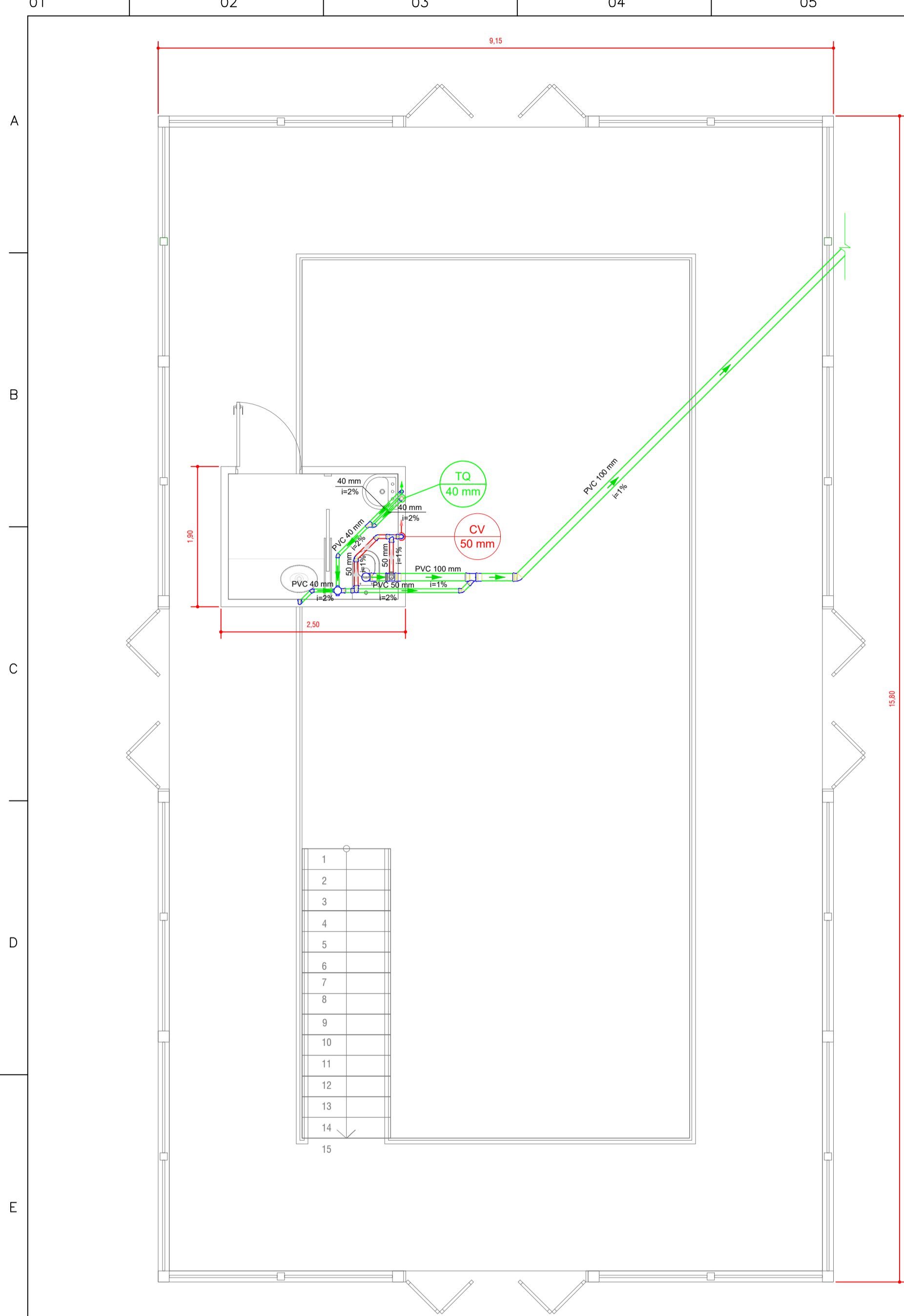
PLANTA BAIXA DO PROJETO DE ESGOTO PAVIMENTO TÉRREO Escala 1:100
