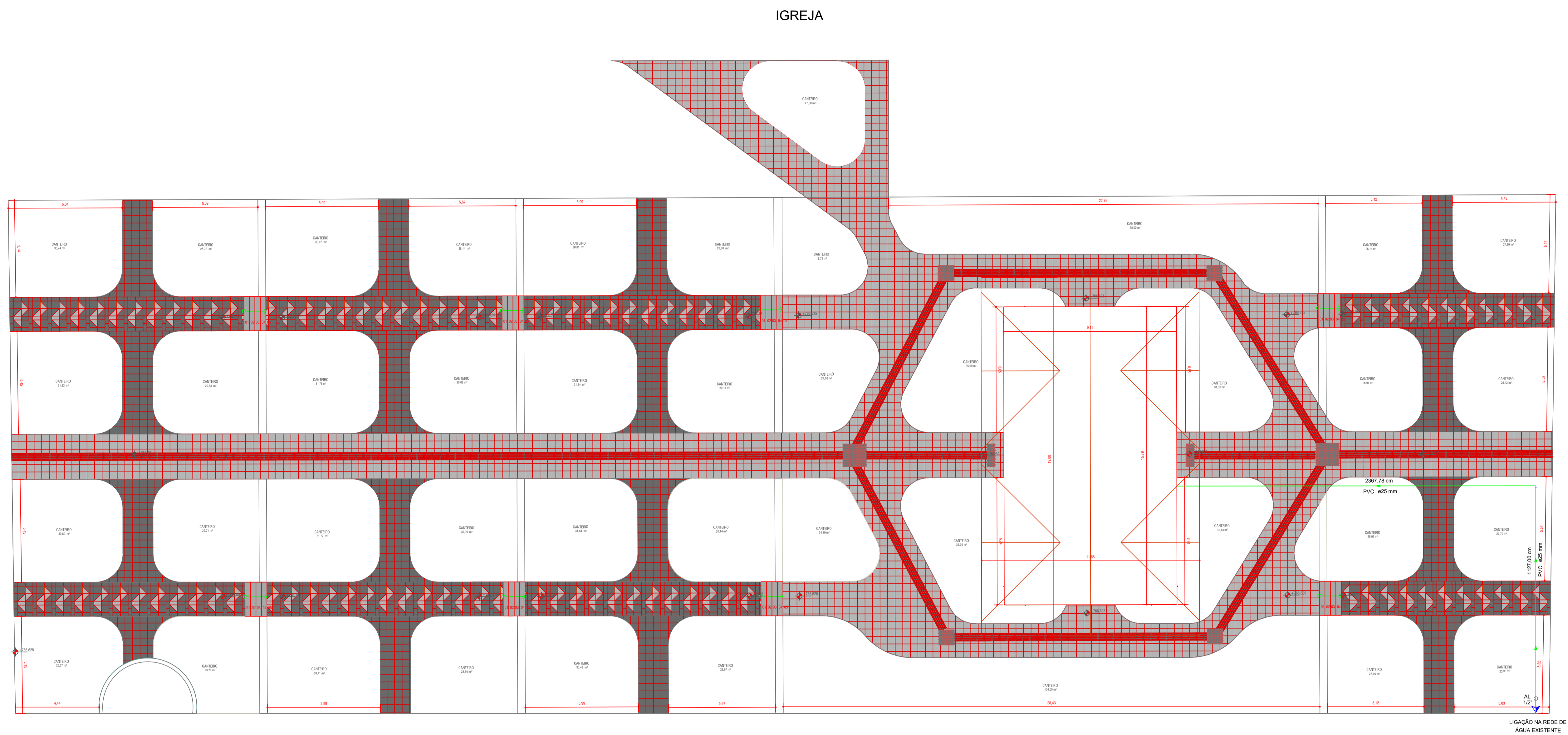
PLANTA DE IMPLANTAÇÃO DA REDE HIDRÁULICA Escala 1:125
