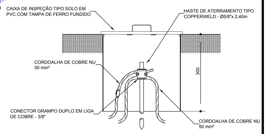
DETALHE CAIXA DE INSPEÇÃO
