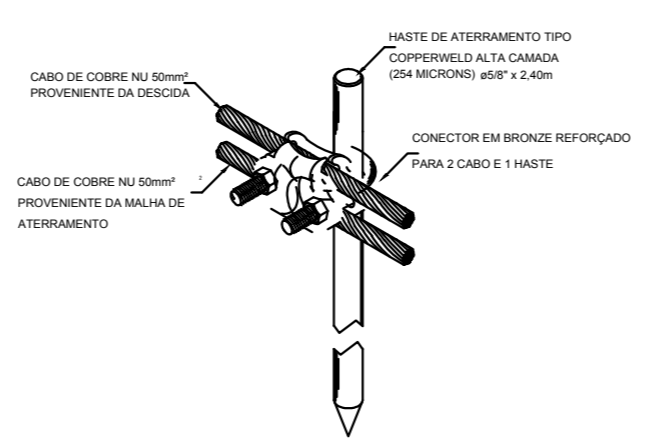
DETALHE DE UTILIZAÇÃO DO CONECTOR NA HASTE DE ATERRAMENTO
