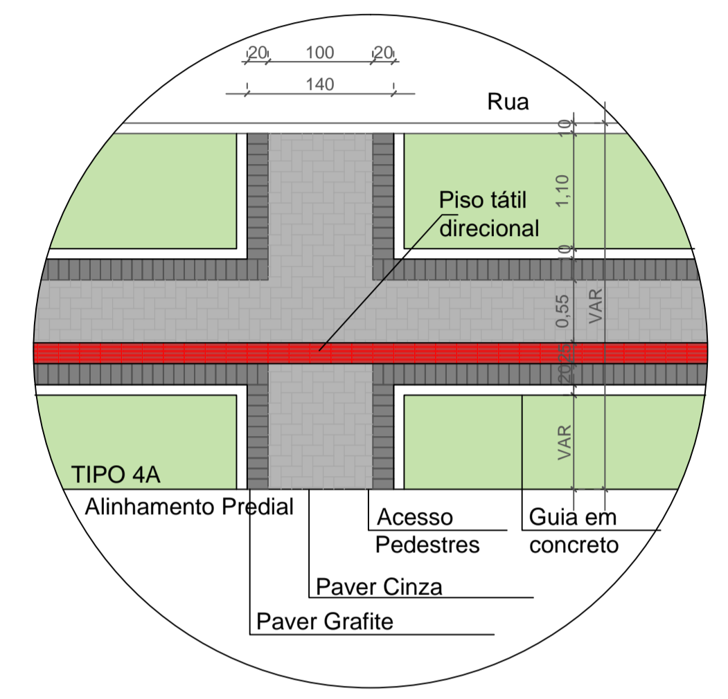
DETALHE RAMPA DE ACESSO Sem escala
