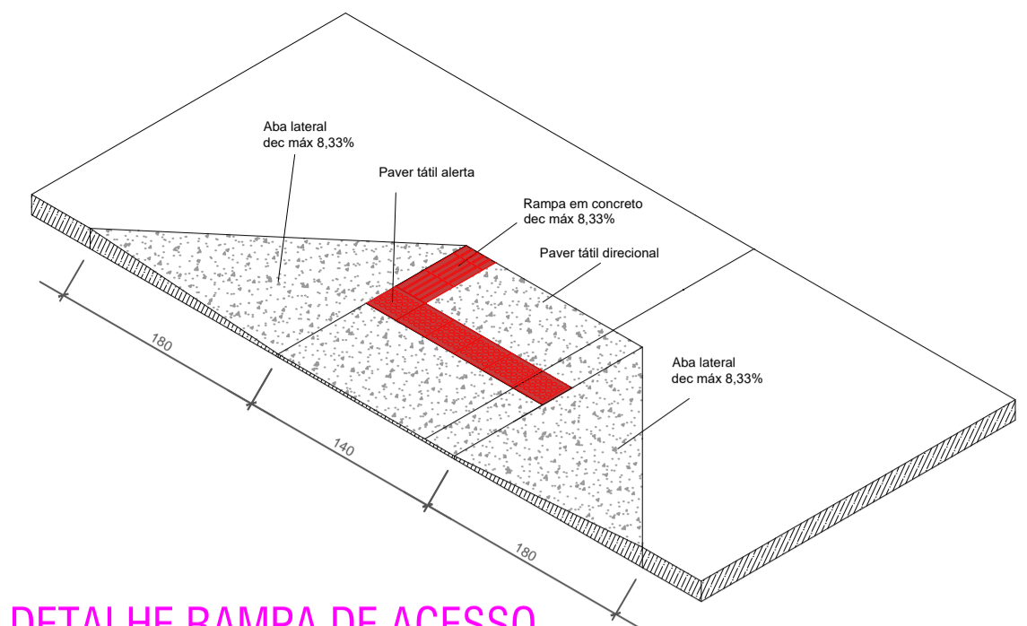
DETALHE RAMPA DE ACESSO Sem escala
