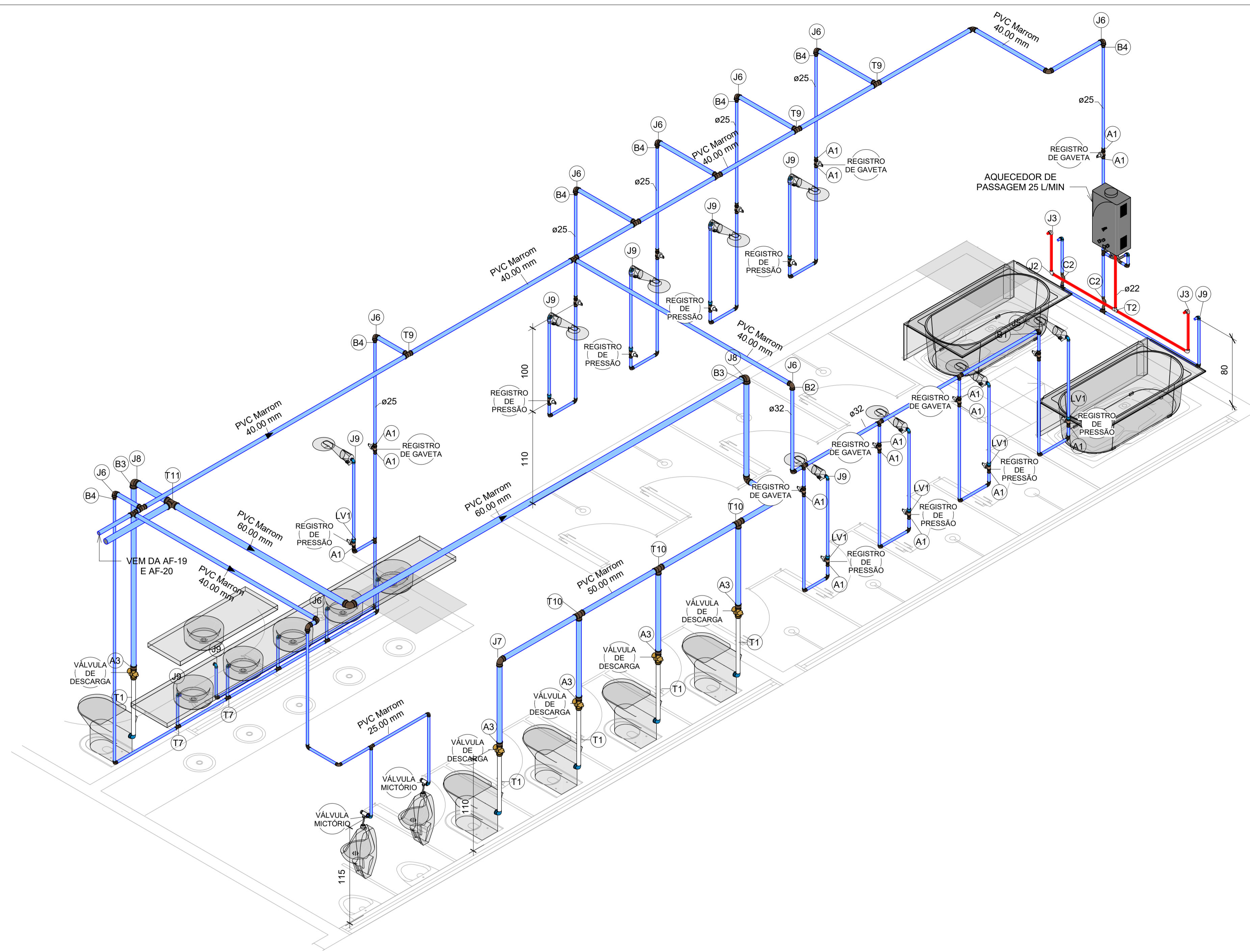
2 DET. VISTA 3D
