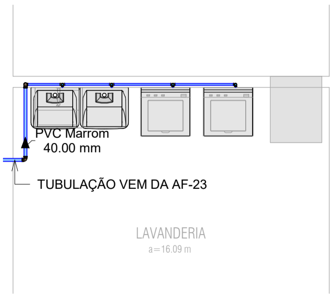
4 DET. PLANTA HIDRÁULICA 1 : 50
