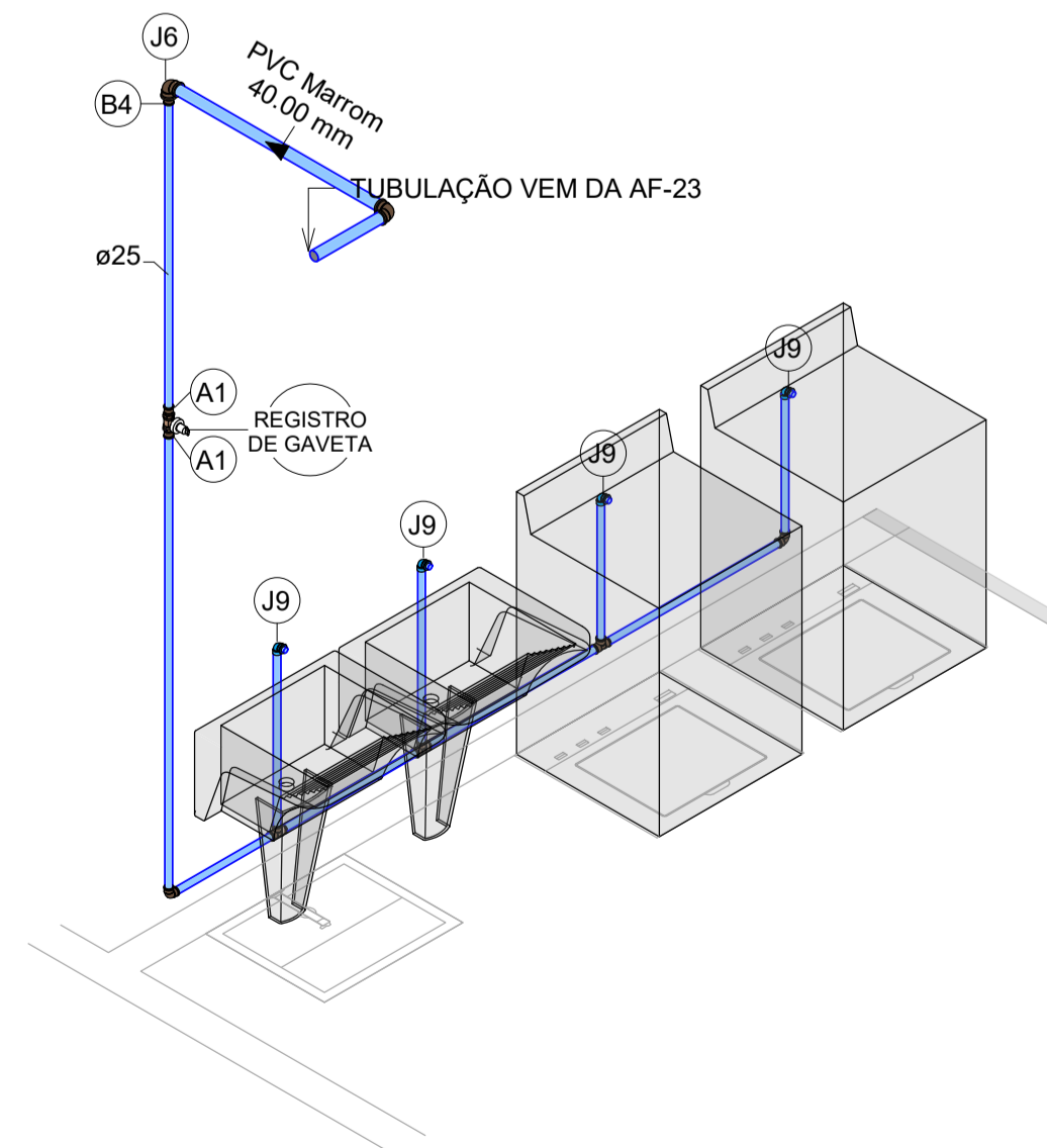
3 DET. VISTA 3D
