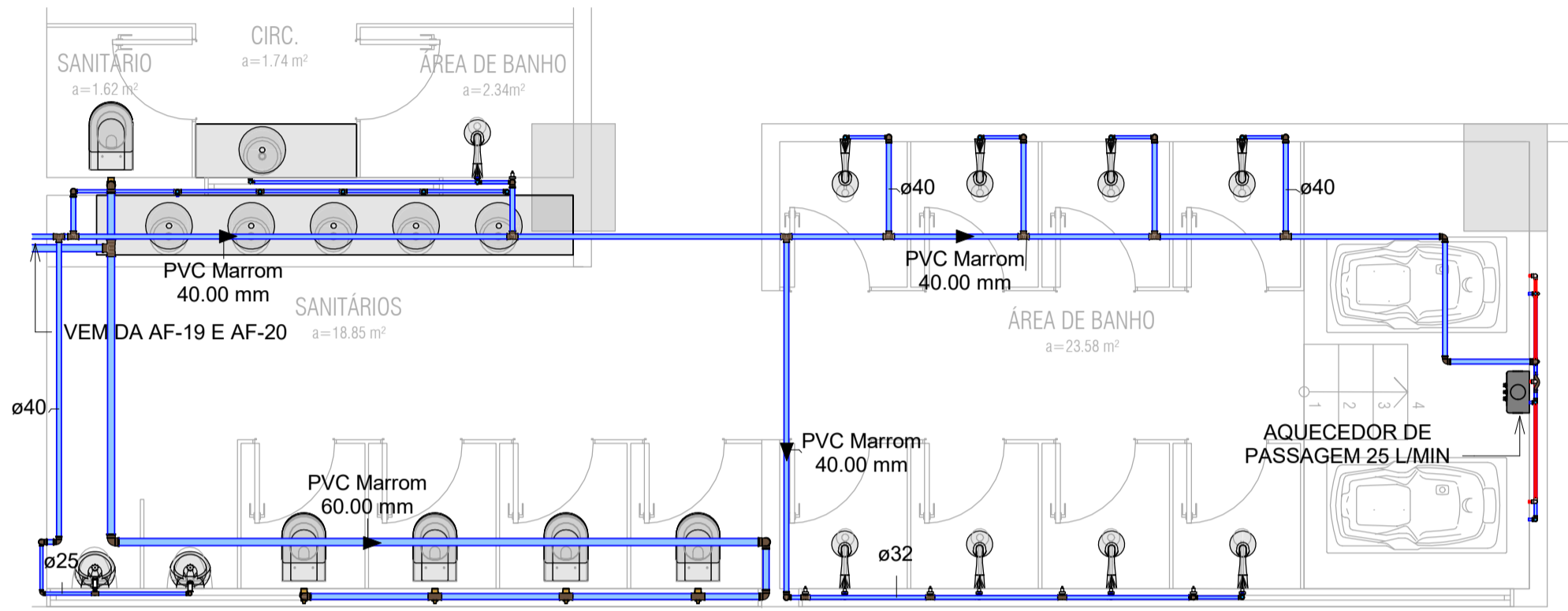
1 DET. PLANTA HIDRÁULICA 1 : 50
