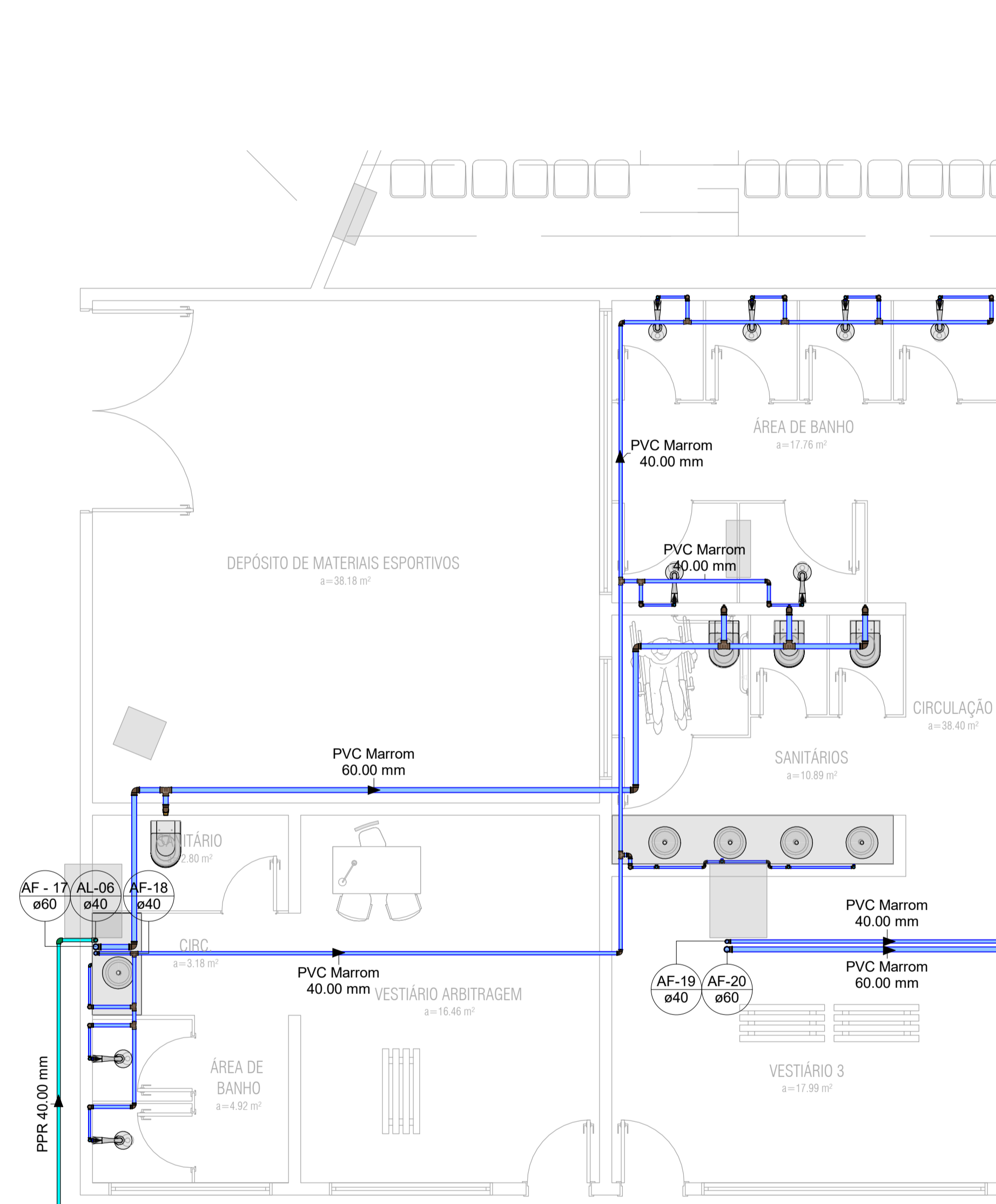
1 DET. PLANTA HIDRÁULICA 1:50
