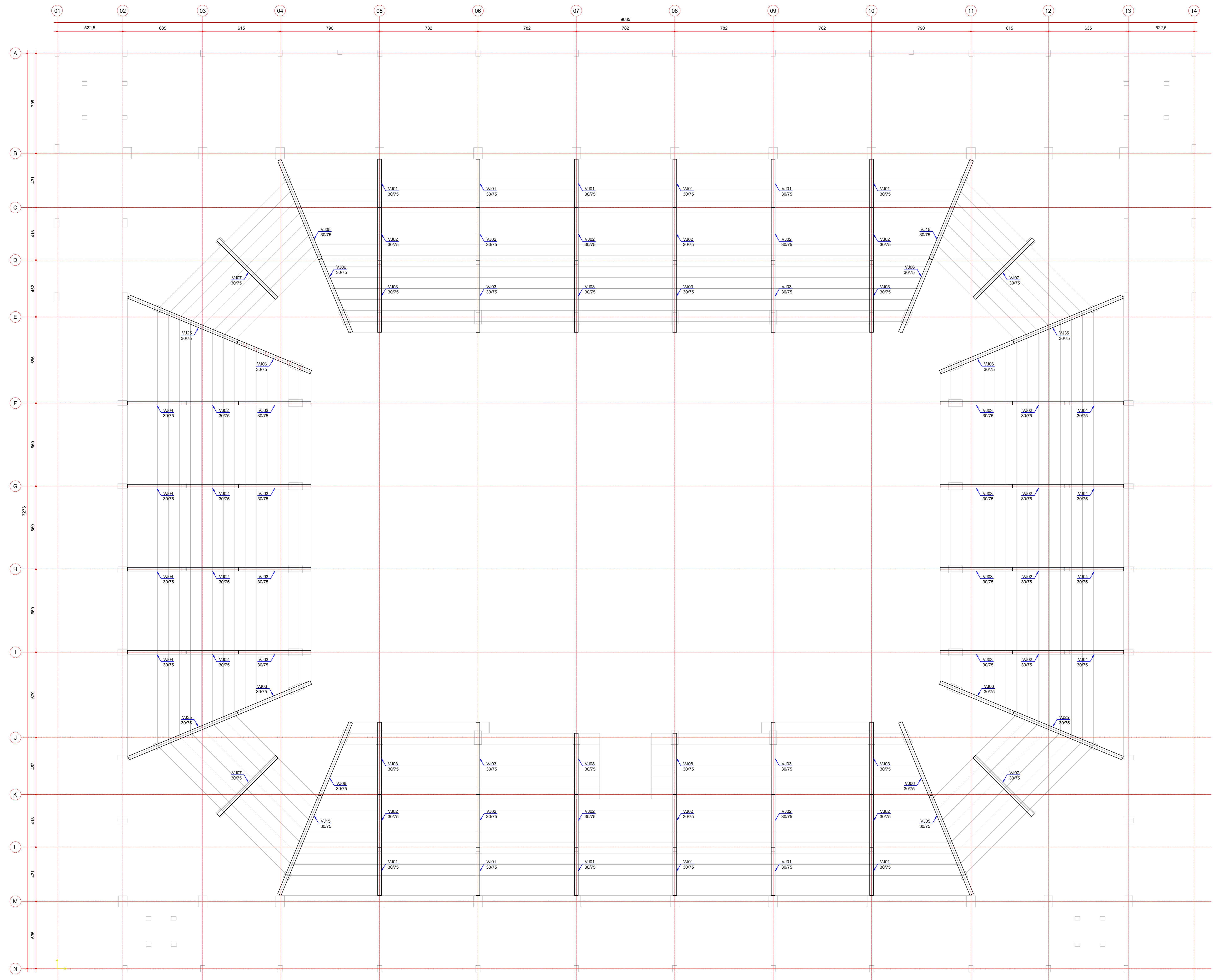
PLANTA DE LOCAÇÃO - VIGAS JACARÉ ESCALA: 1:725
