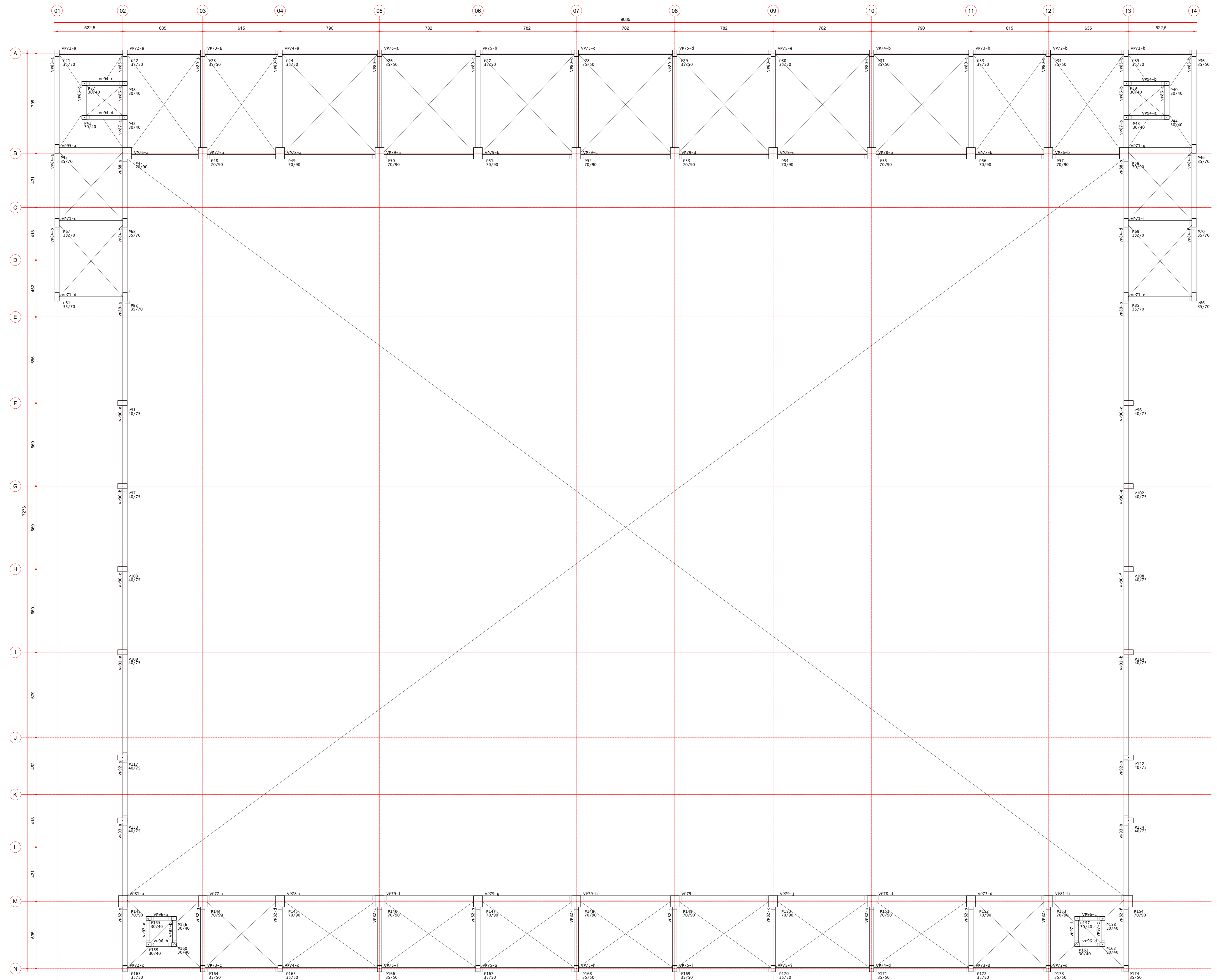
PLANTA DE LOCAÇÃO - SEGUNDO PAVIMENTO ESCALA: 1:125
