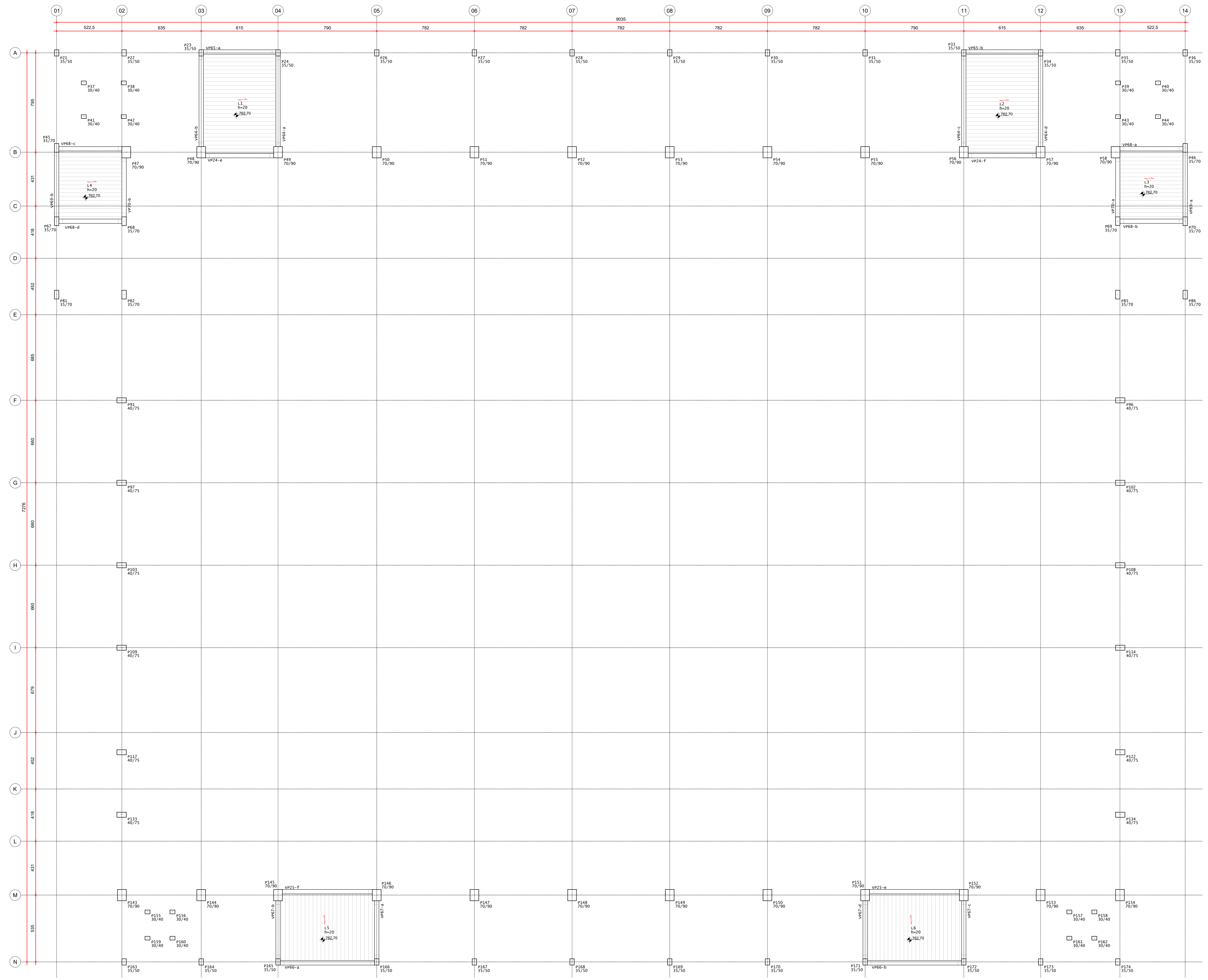
PLANTA DE LOCAÇÃO - LAJE TÉCNICA 02 ESCALA: 1:125
