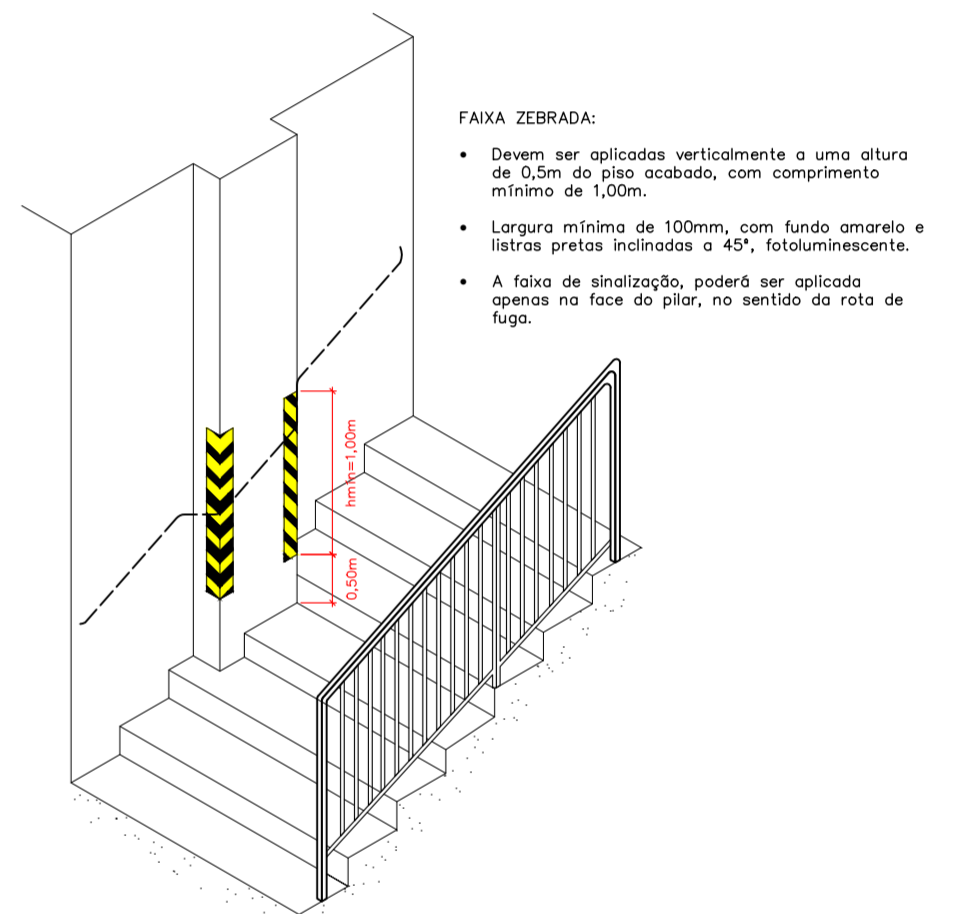
DETALHE: SINALIZAÇÃO COMPLEMENTAR EM OBSTÁCULOS ESCALA= SEM ESCALA
