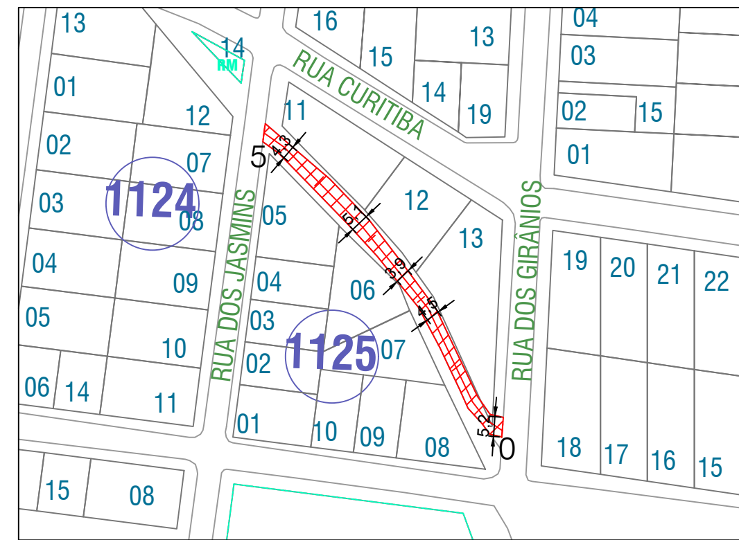
PAVIMENTO EXISTENTE - RUA DARCY GOMES BRASIL Esc. 1/750
