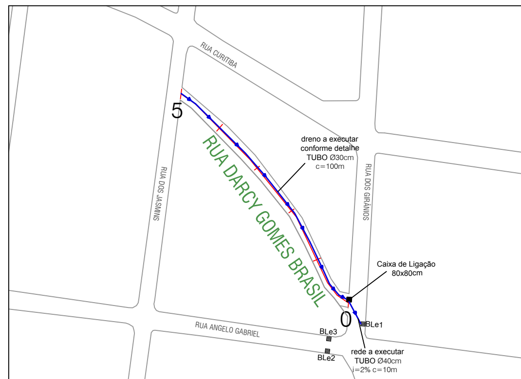
DRENAGEM E MEIO-FIO - RUA DARCY GOMES BRASIL Esc. 1/750
