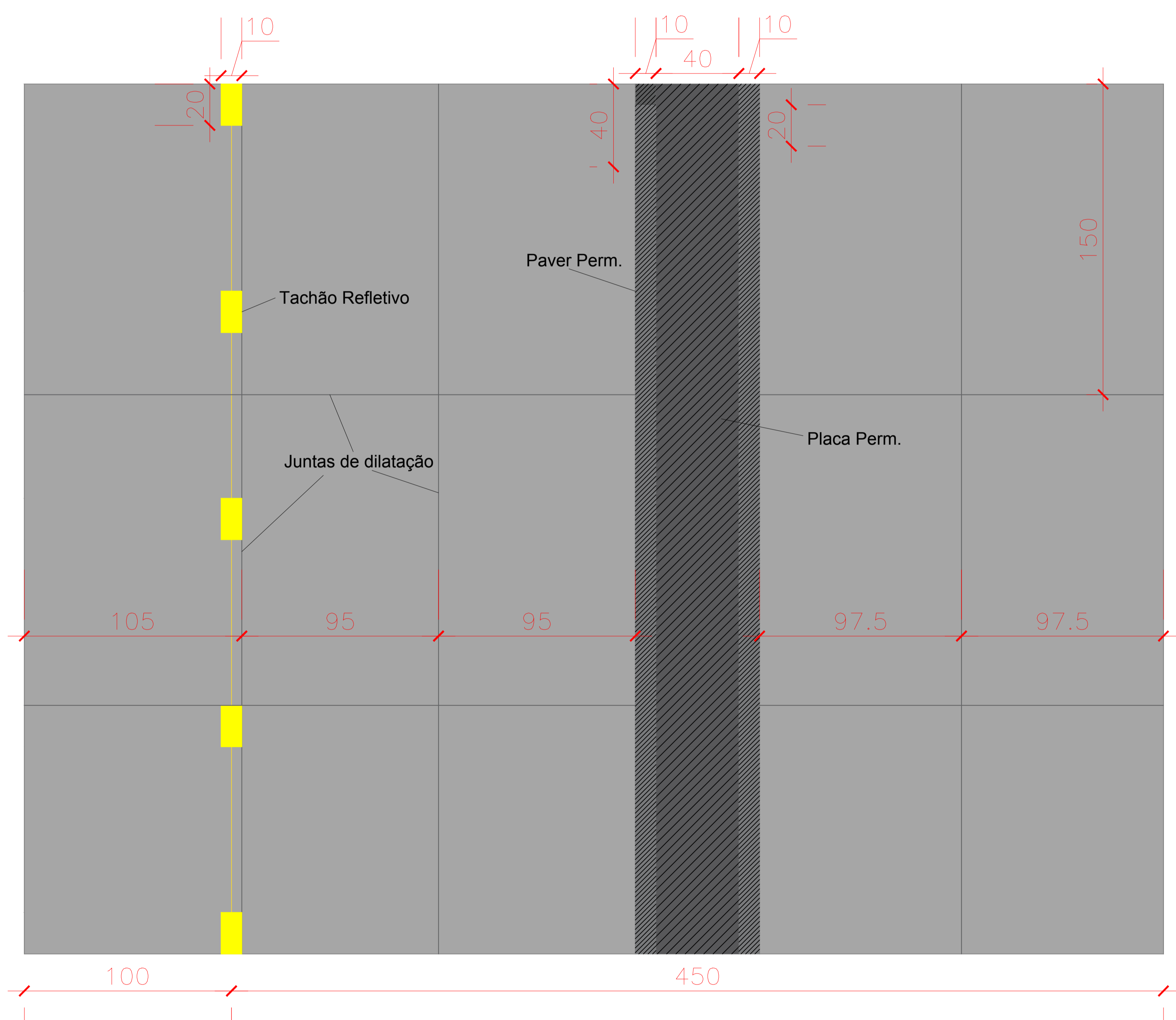
PLANTA BAIXA DA RUA COM JUNTAS DE DILATAÇÃO, DRENAGEM E TACHÃO MEDIDAS EM CM SEM ESCALA
