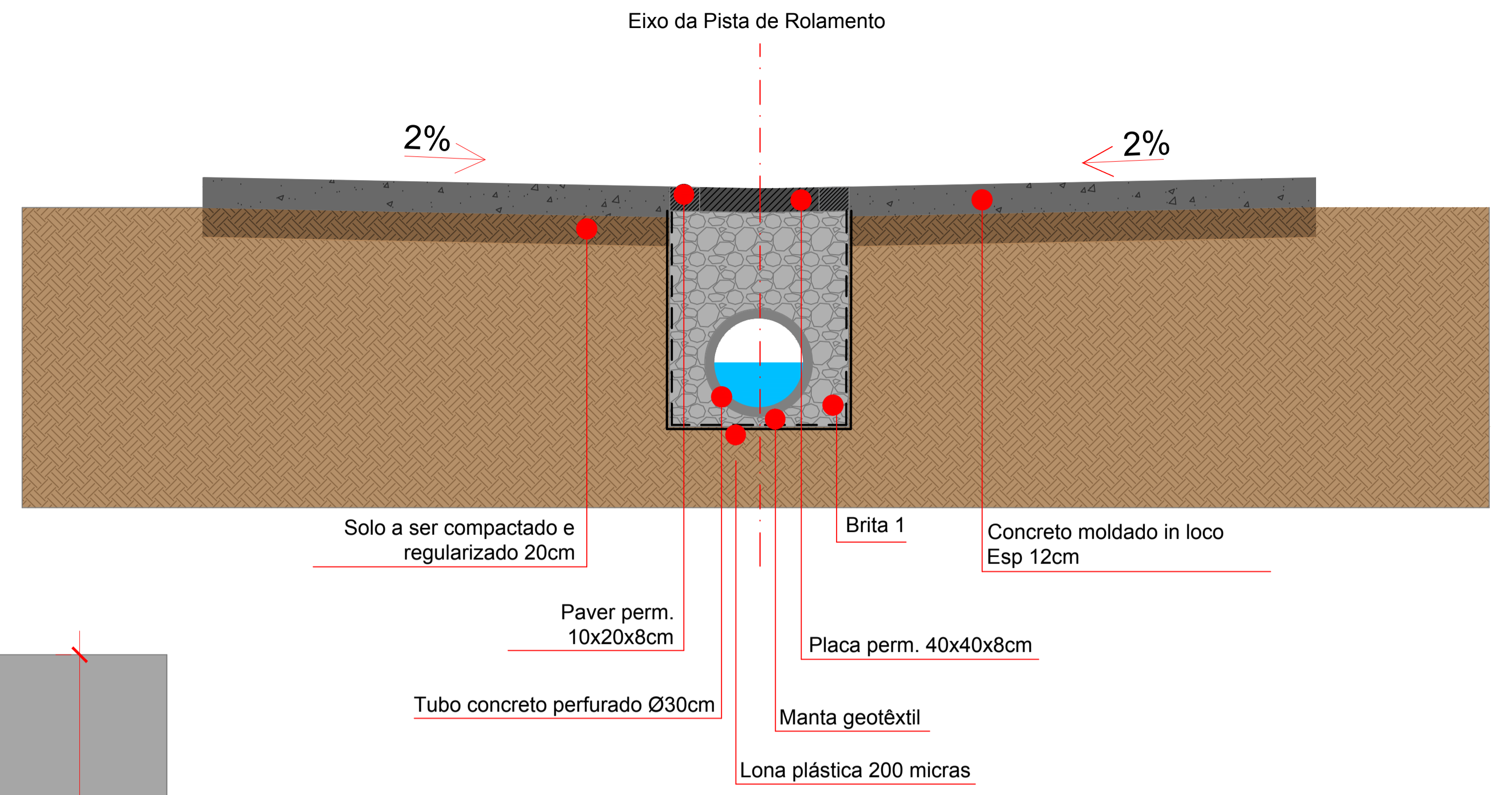
DETALHES DRENAGEM - CORTE GENÉRICO MEDIDAS EM CM SEM ESCALA
