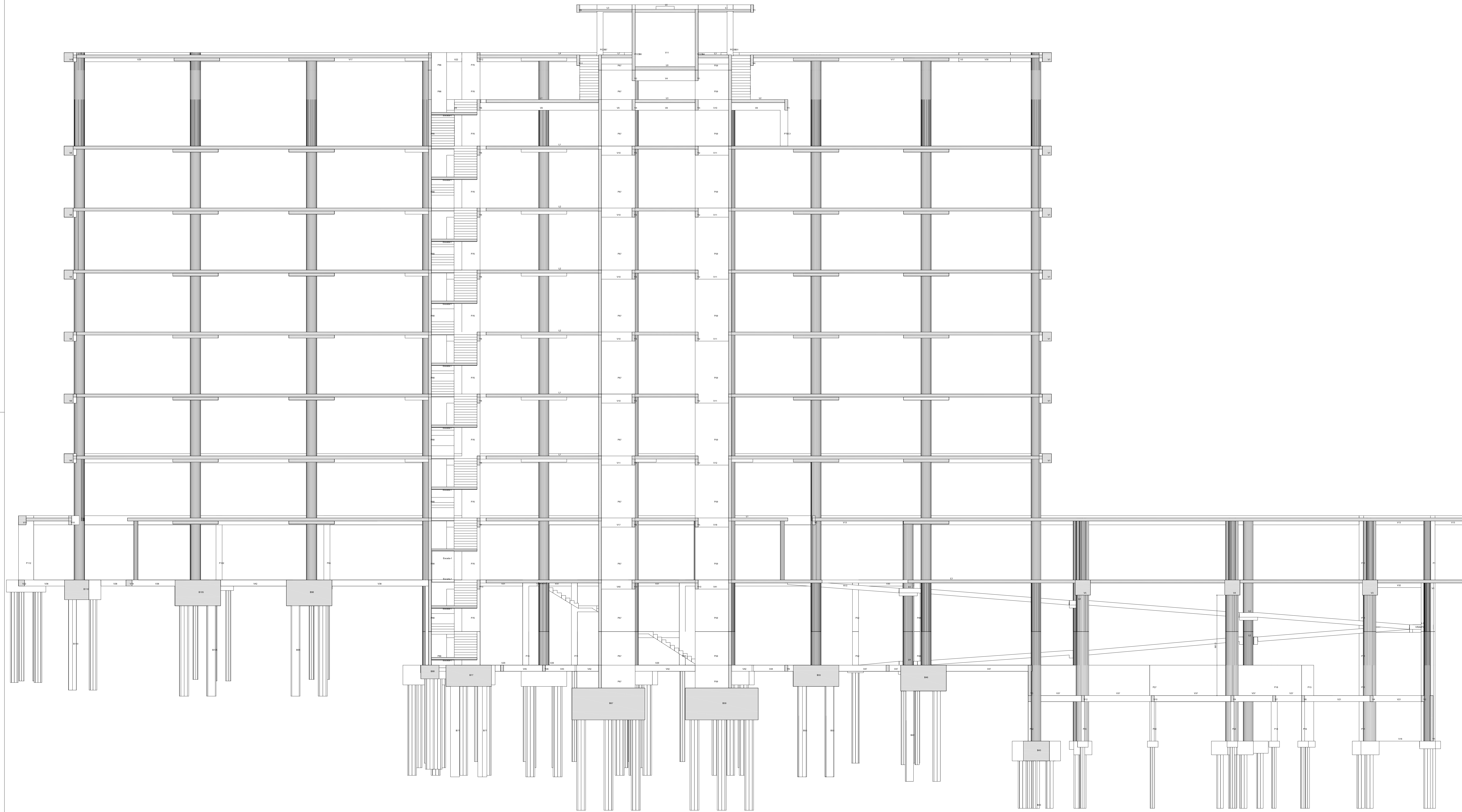
CORTE LONGITUDINAL
