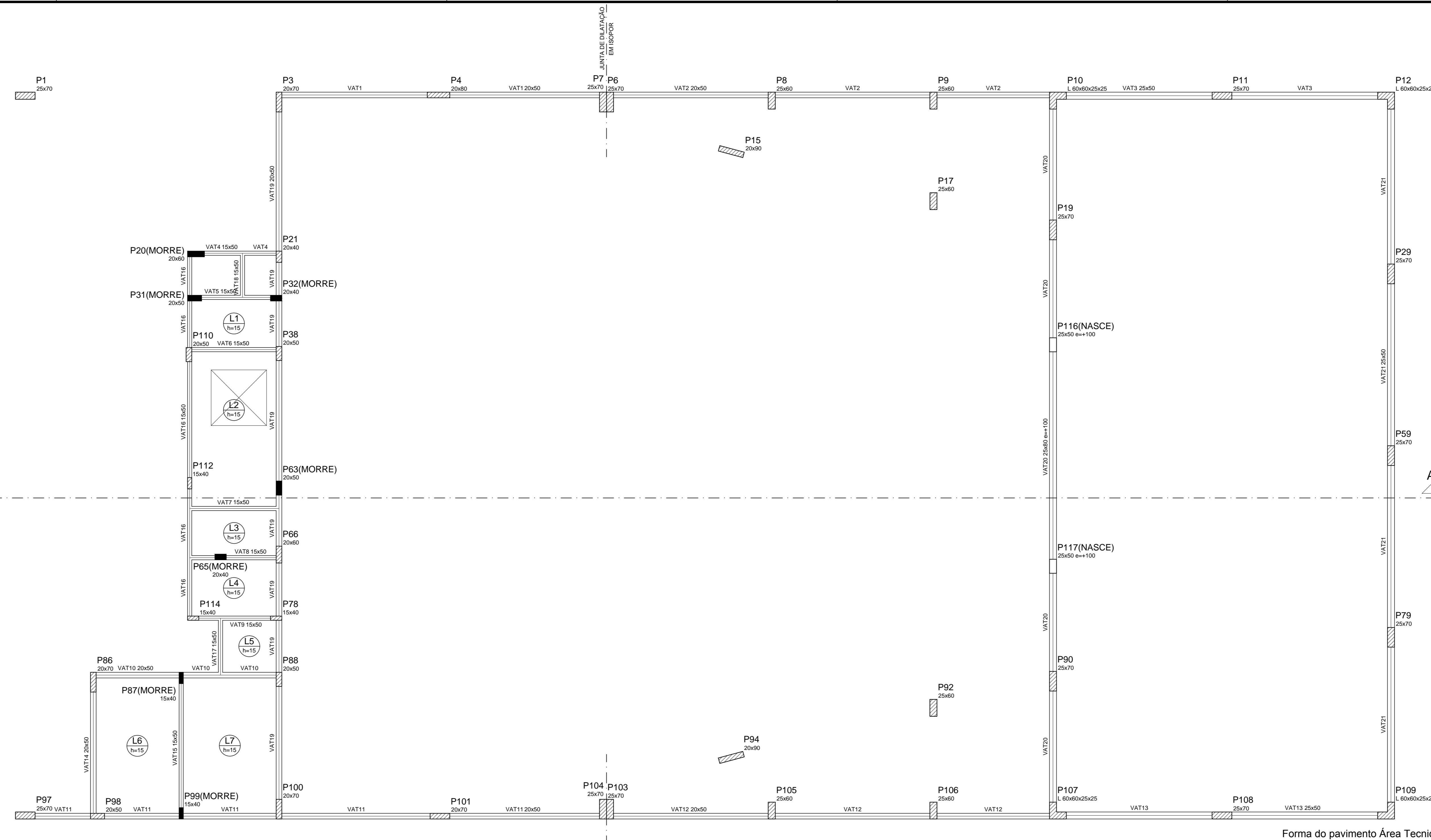
Forma do pavimento Área Técnica escala 1:75
