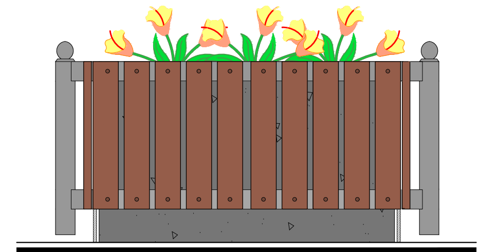
VISTA LATERAL - FLOREIRA ESC: 1/10
