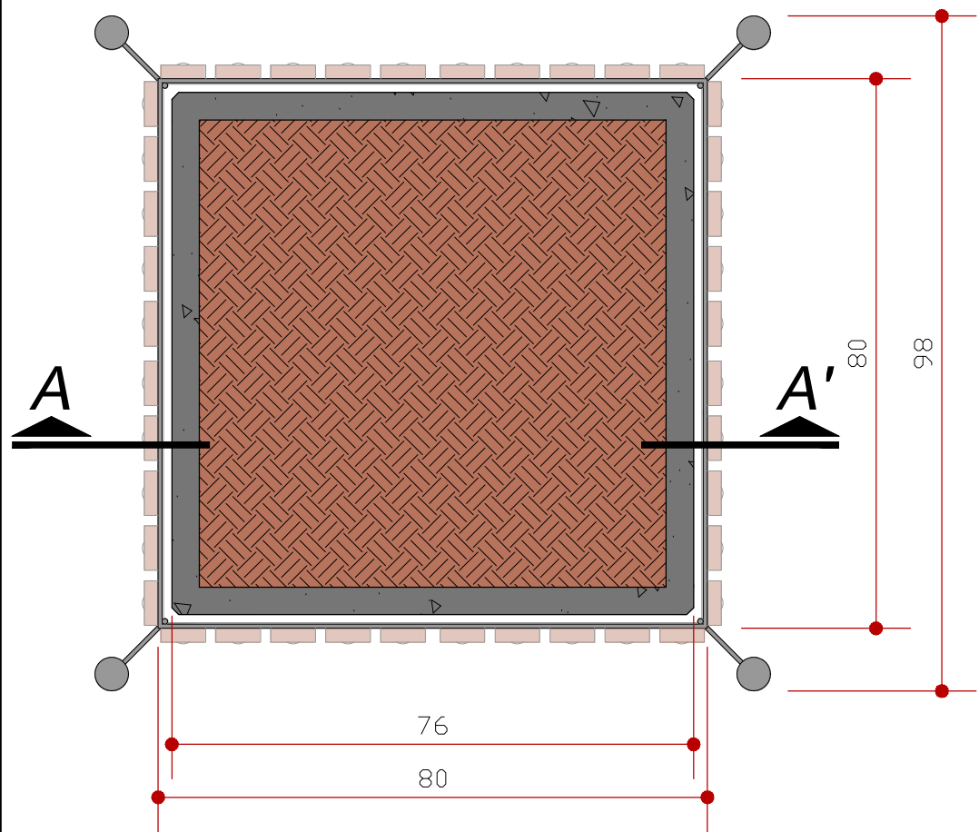
PLANTA BAIXA - FLOREIRA + CAIXA DE CONCRETO
